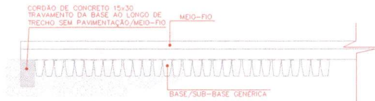
CORTE DETALHE CORDÃO EM CONCRETO
