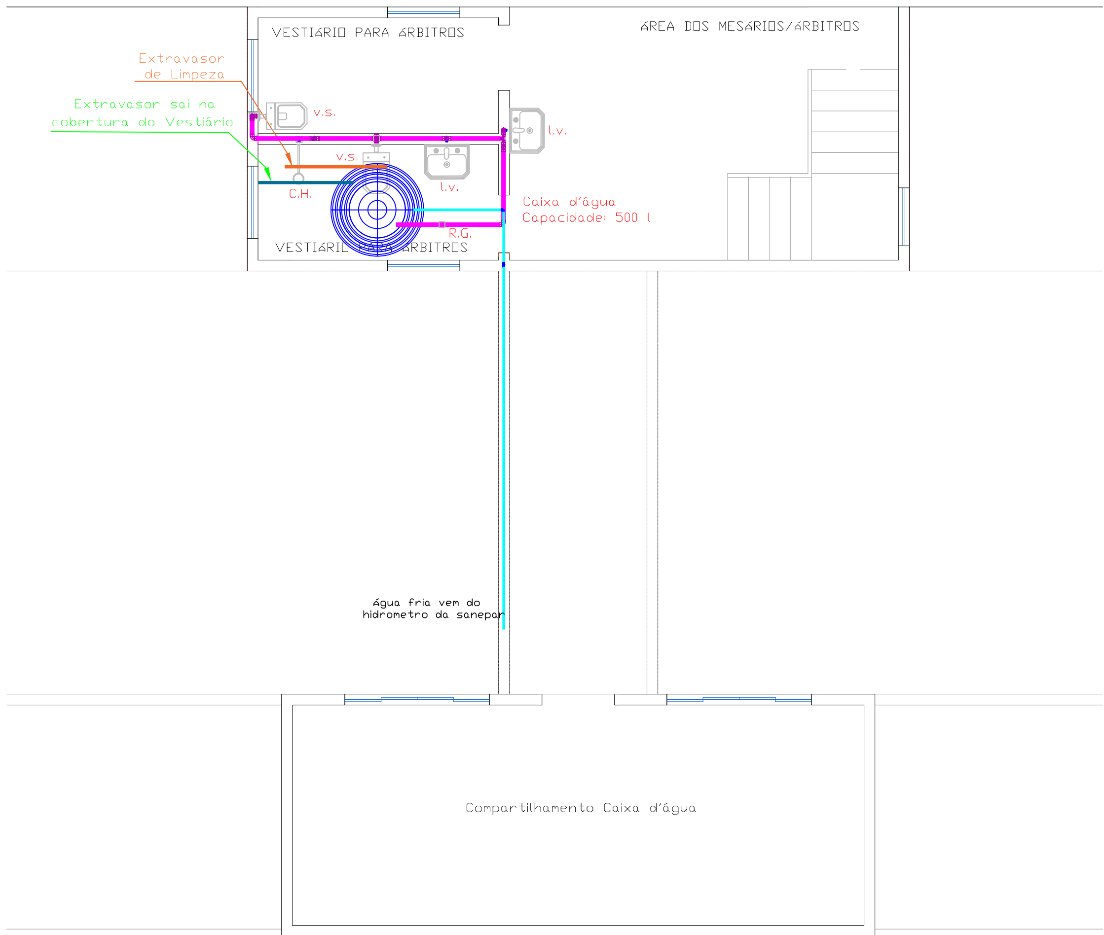
PLANTA BAIXA - 2º PAVIMENTO TUBULAÇÕES DE ÁGUA FRIA ESCALA: 1/50
