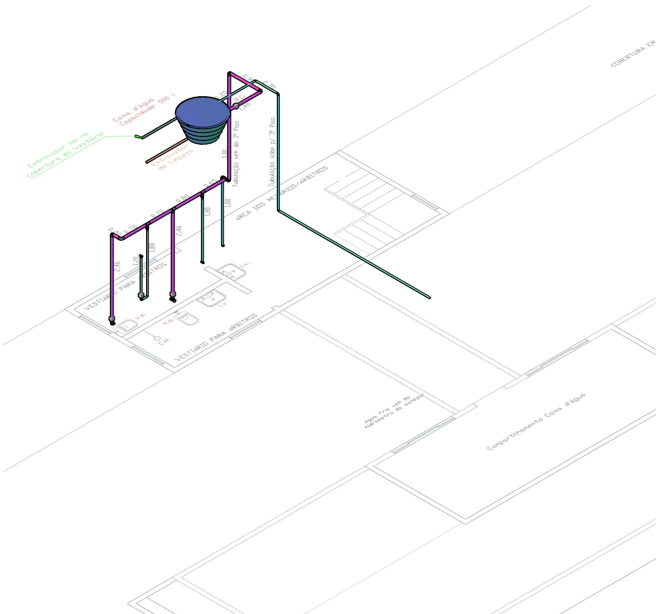
PLANTA BAIXA ISOMÉTRICA - 2º PAVIMENTO TUBULAÇÕES DE ÁGUA FRIA ESCALA: 1/50
