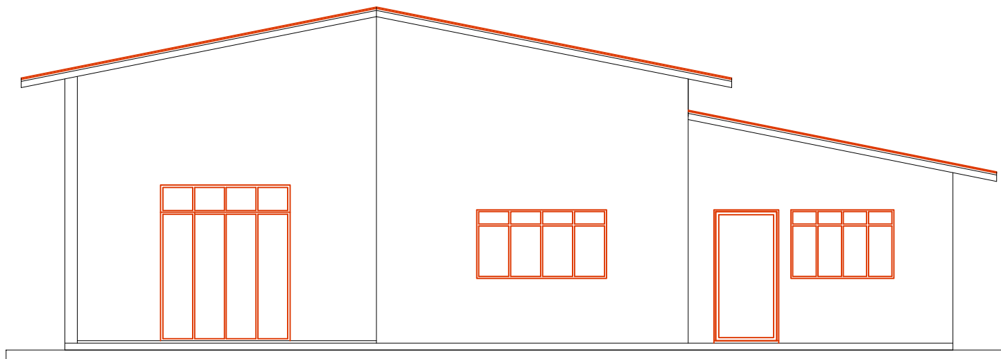
ELEVAÇÃO FRONTAL
