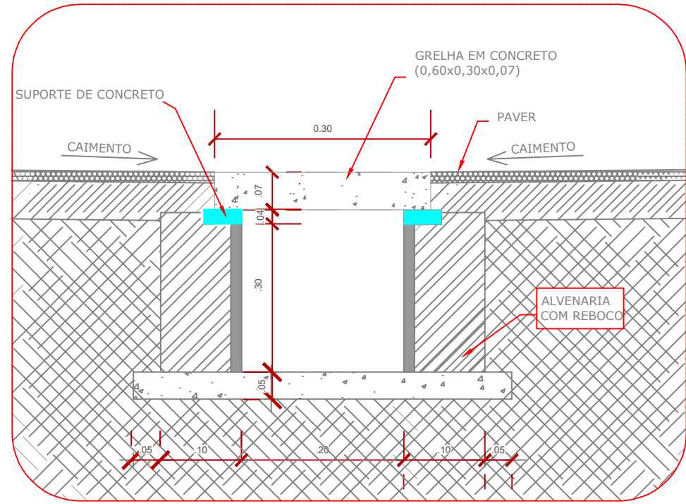
4 DETALHE CANALETA SEM ESCALA
