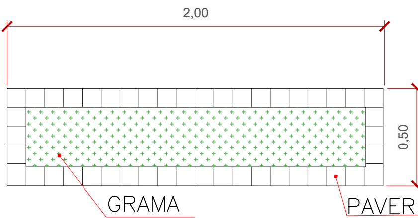
3 DETALHE CANTEIRO ESC 1:20
