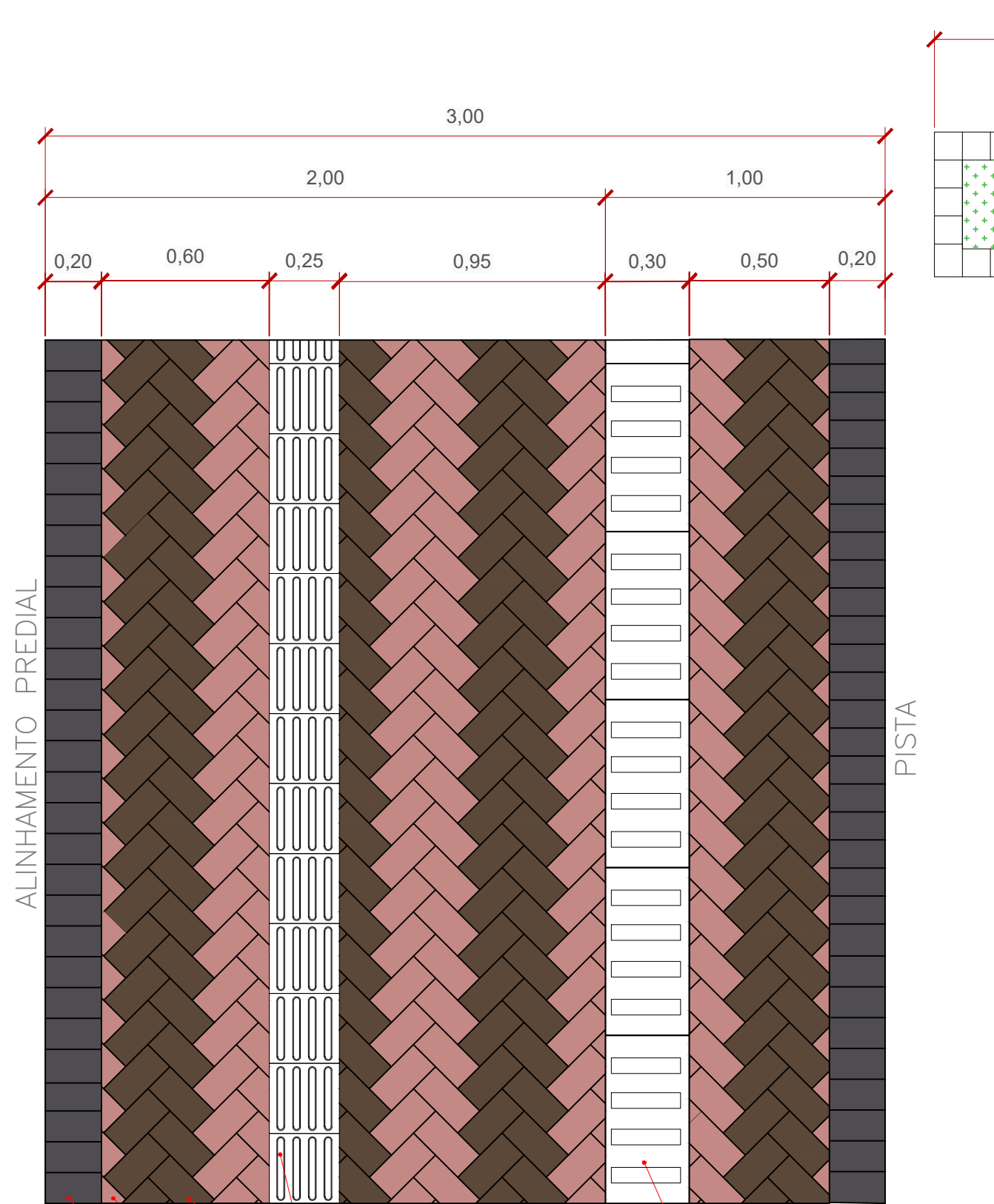
3 DETALHE CANTEIRO ESC 1:20
