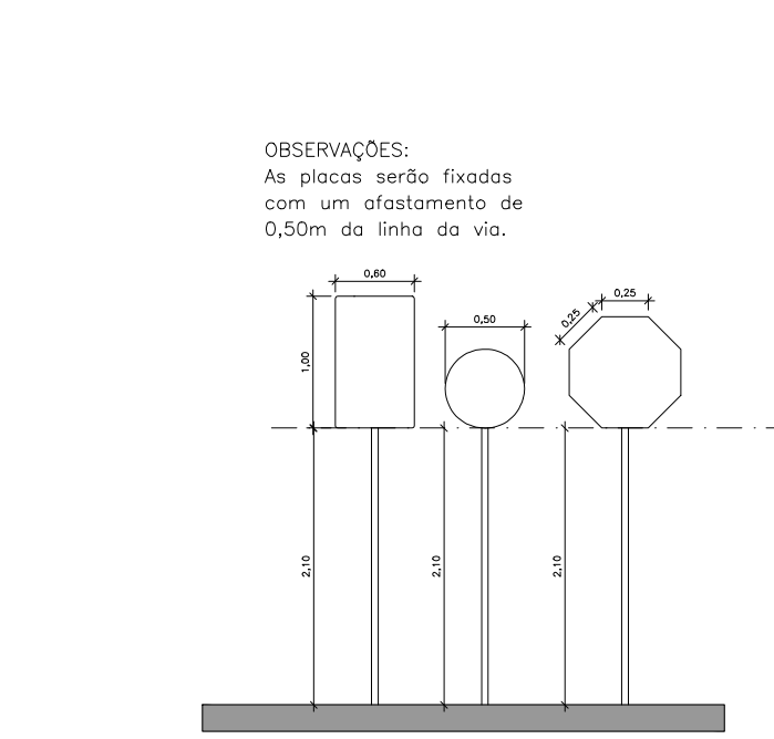
3 - DETALHE ASSENTAMENTO DAS PLACAS ESC:1/50
