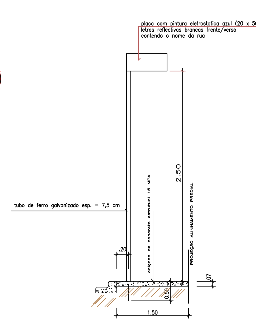
2 - DETALHE DA PLACA NOME DAS RUAS ESC 1/50
