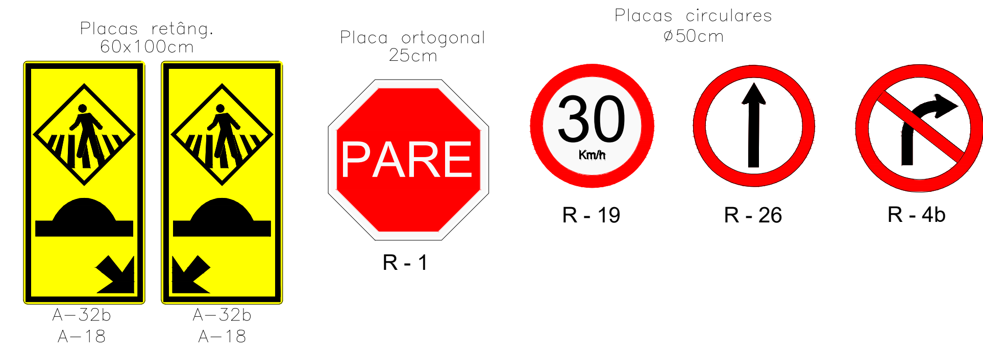
1 - DETALHE DAS PLACAS ESC:1/25
