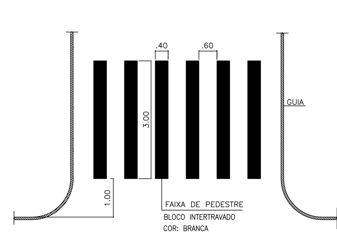
5 - DETALHE FAIXA DE PEDESTRES SEM ESCALA
