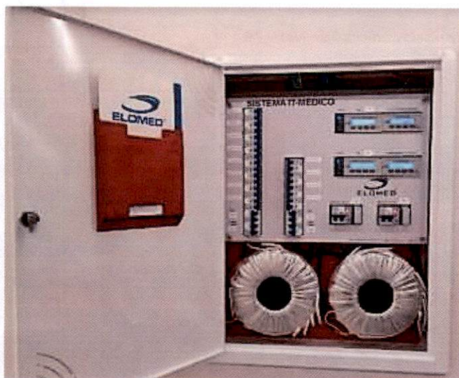
← Imagem Ilustrativa de dois Sistemas IT Médico em centro de distribuição embutido SIT13000/DT-E.
