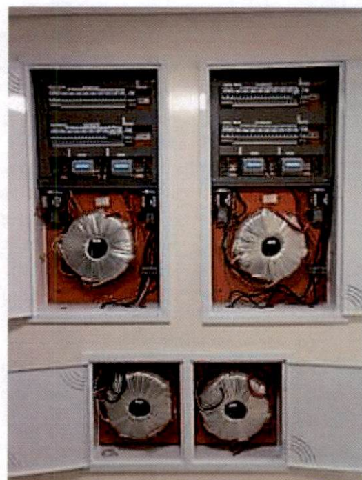
Imagem ilustrativa de quatro Sistemas IT Médico em centro de distribuição embutido SIT14000/DT-E e SIT14000/TE. →
