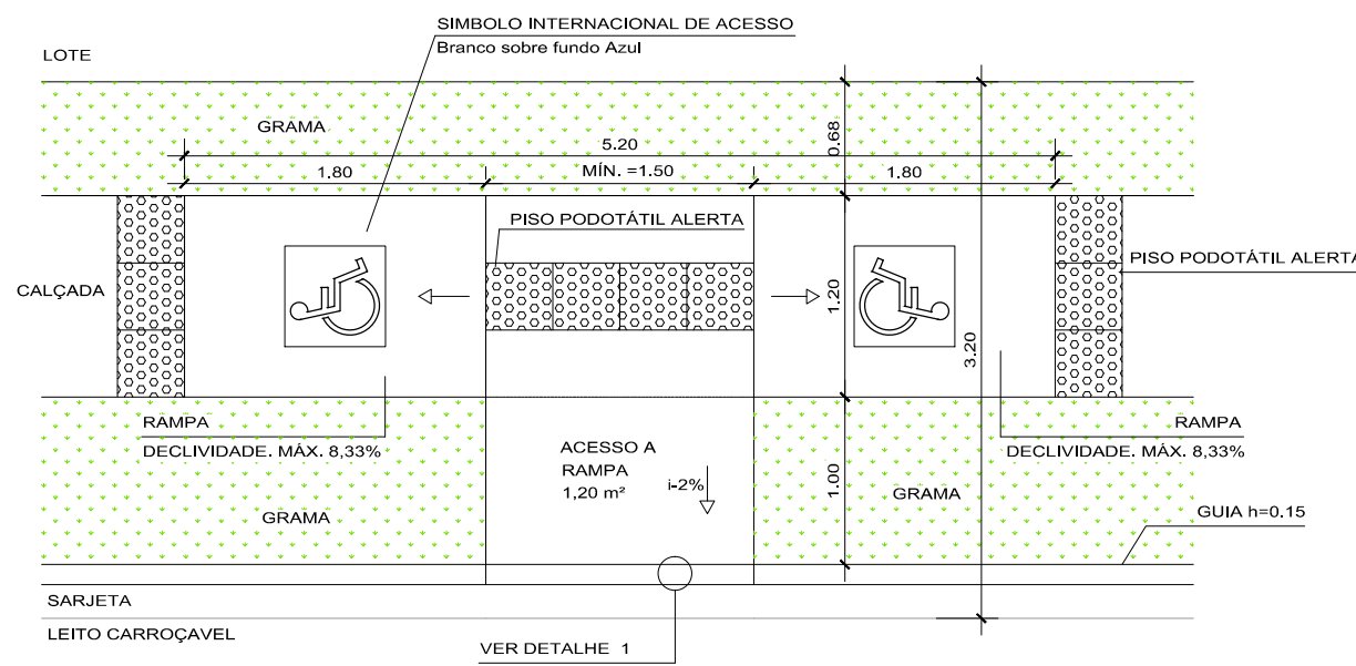
DETALHE RAMPA ACESSIBILIDADE PASSEIO - 3,20m
