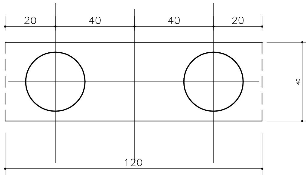
PLANTA
