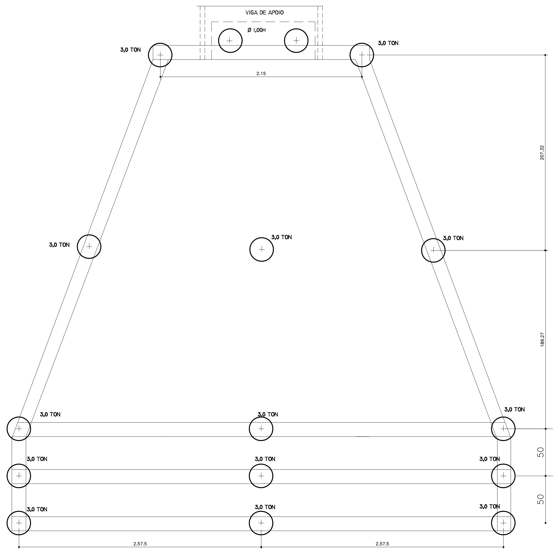
LOCAÇÃO DAS ESTACAS
