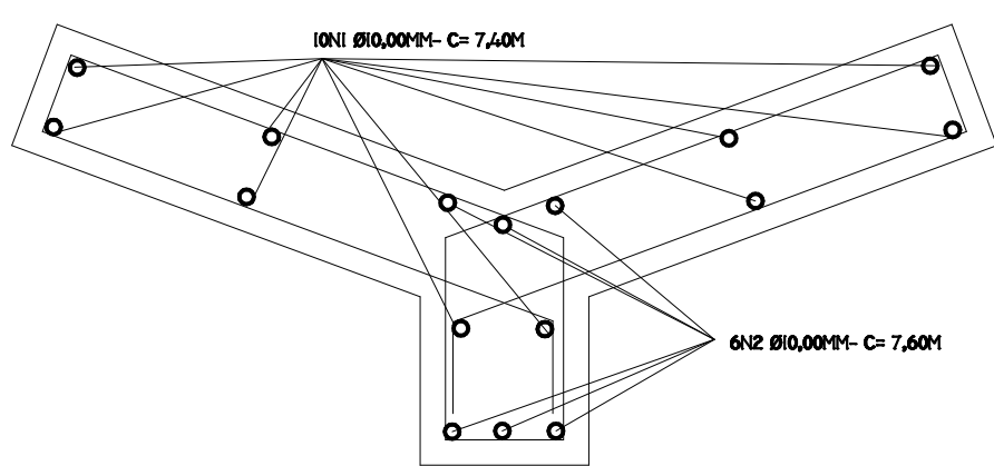
ARMADURA
