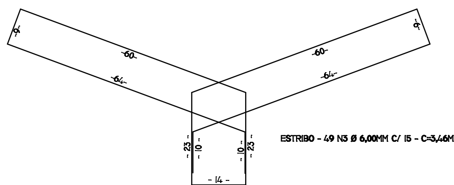
ARMADURA
