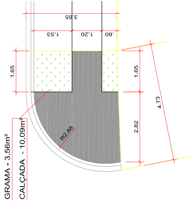
DETALHE - SETOR S01
