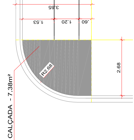
DETALHE - SETOR S03
