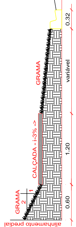
DETALHE PASSEIO COM DESNIVEL
