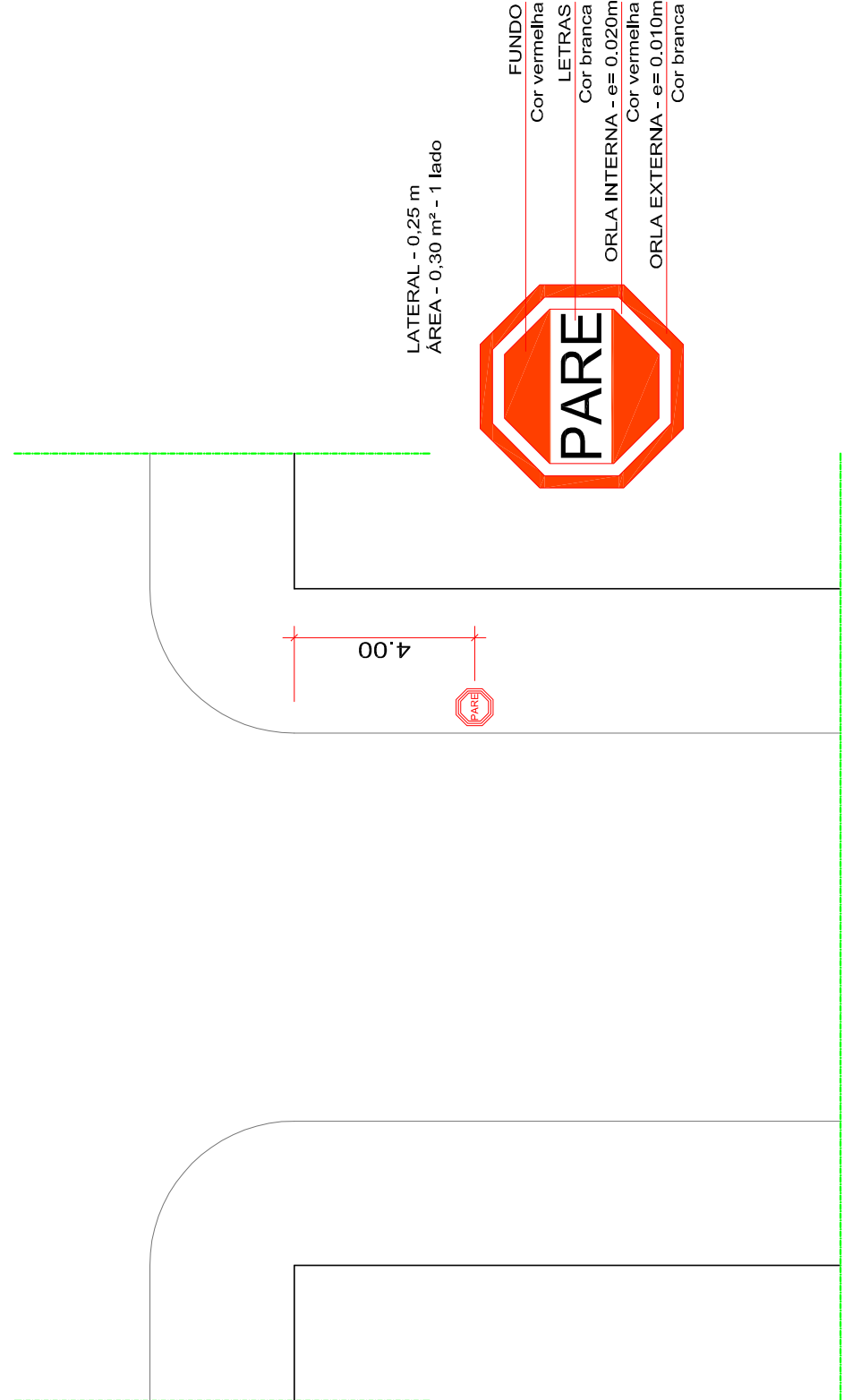
DETALHE SINALIZAÇÃO VERTICAL SINALIZAÇÃO VIÁRIA ESCALA 1:200
