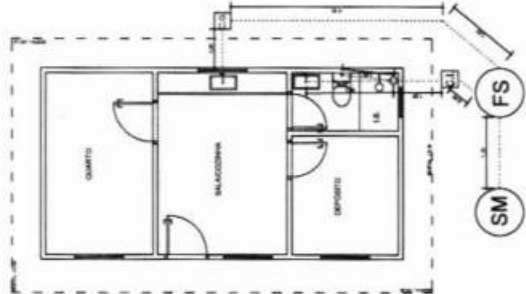
PLANTA BAIXA - HIDROSSANITÁRIO ESC.: 1/75
