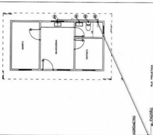
PLANTA BAIXA - ÁGUA FRIA ESC.: 1/75
