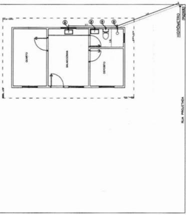
PLANTA BAIXA - ÁGUA FRIA ESC.: 1/75
