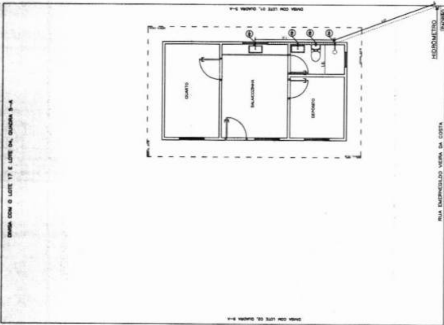
PLANTA BAIXA - ÁGUA FRIA ESC.: 1/75
