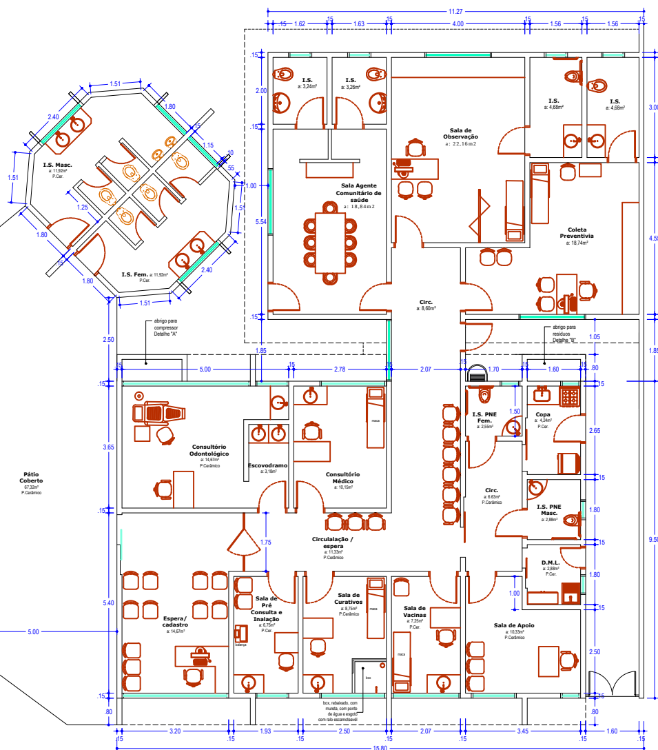
PLANTA BAIXA GERAL (existente e ampliação) Esc.: 1:50
