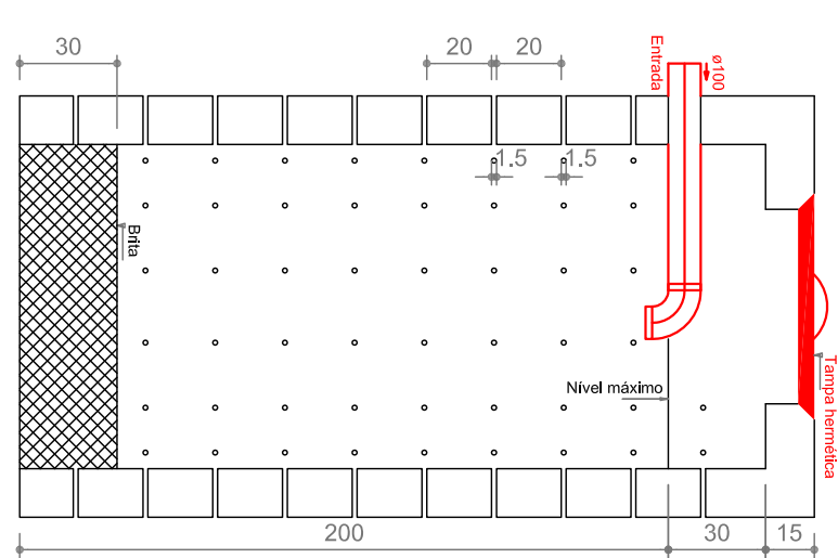
SUMIDOURO CORTE - SEM ESC.
