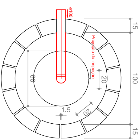
SUMIDOURO PLANTA BAIXA - SEM ESC.
