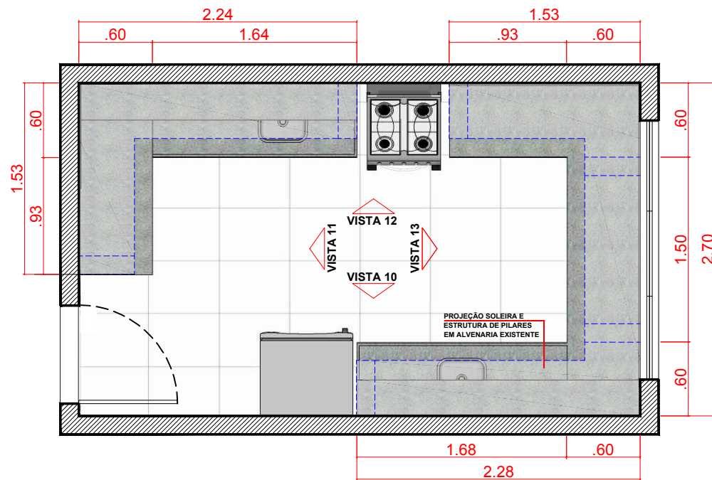
PLANTA BAIXA COZINHA LACTÁRIO CMEI NIL PEREIRA (ANEXO 2)
