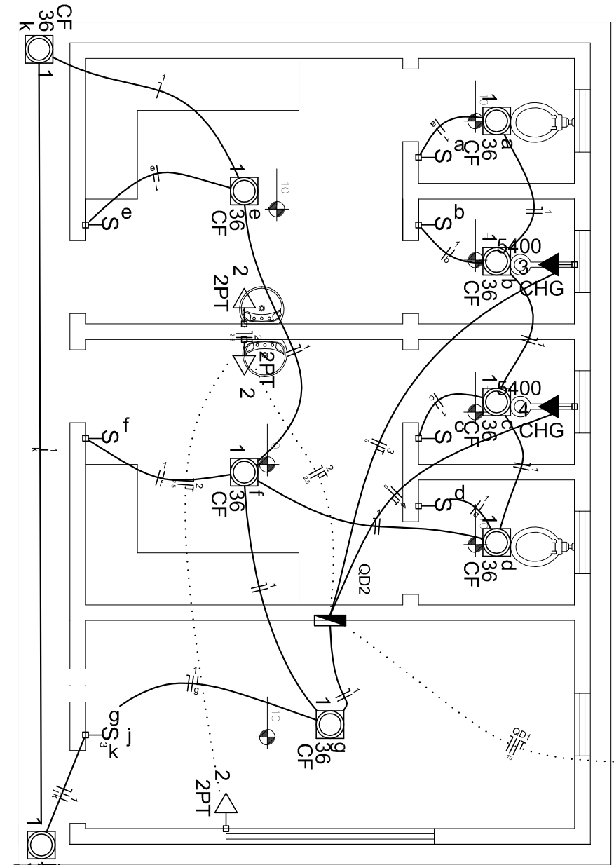
PLANTA BAIXA VESTIARIO ARBITROS
