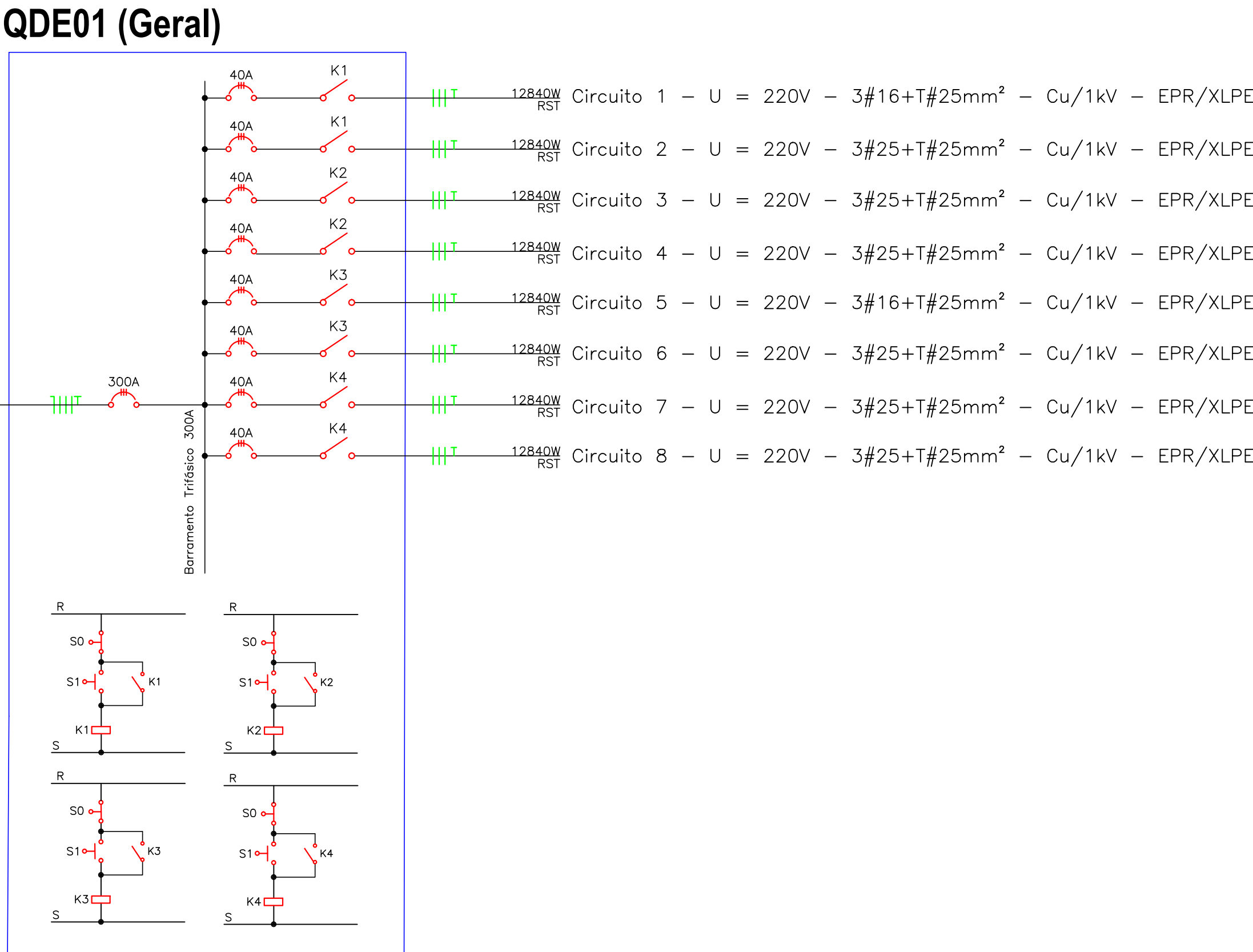
Diagrama unifilar Sem Escala
