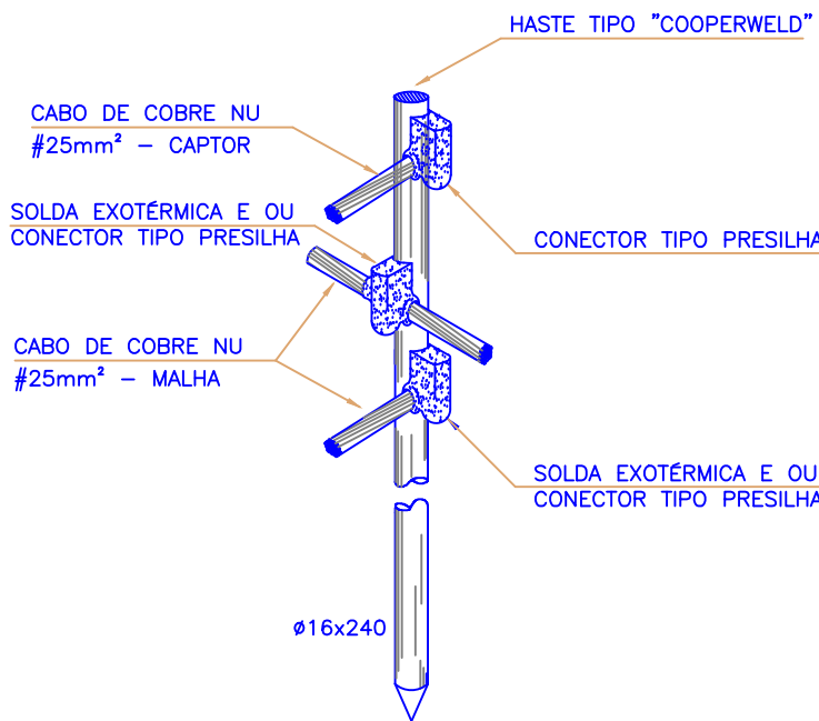
Detalhe haste terra Sem Escala
