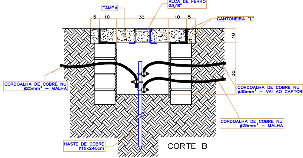
Caixa de passagem Sem Escala
