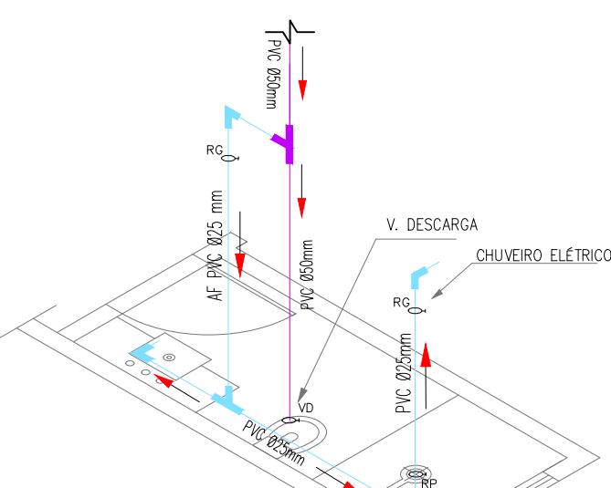
DET. ISOMÉTRICO ÁGUA FRIA 01 e 02 escala: 1/50
