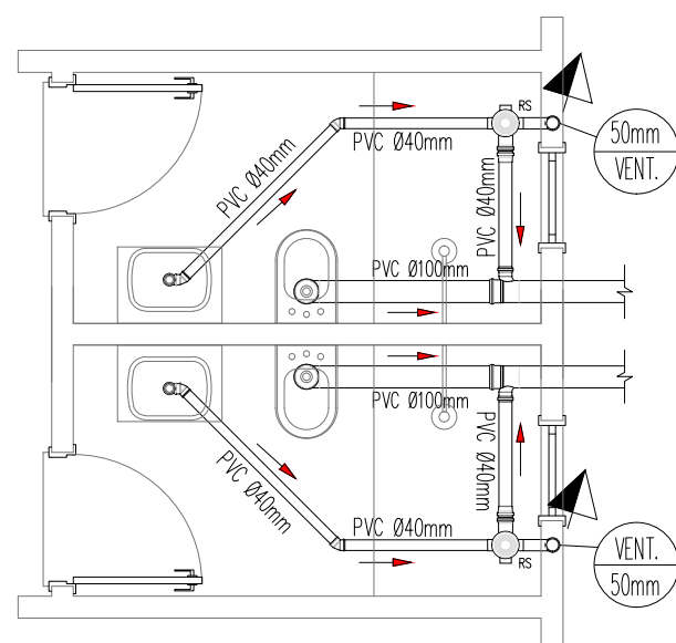
DET. ESGOTO SANITÁRIO 02 escala: 1/50
