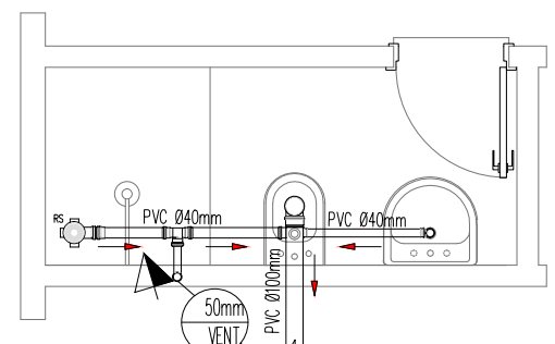
DET. ESGOTO SANITÁRIO 03 escala: 1/50
