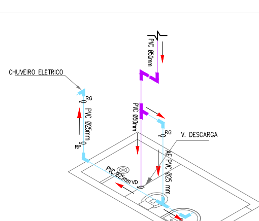
DET. ISOMÉTRICO ÁGUA FRIA 03 escala: 1/50
