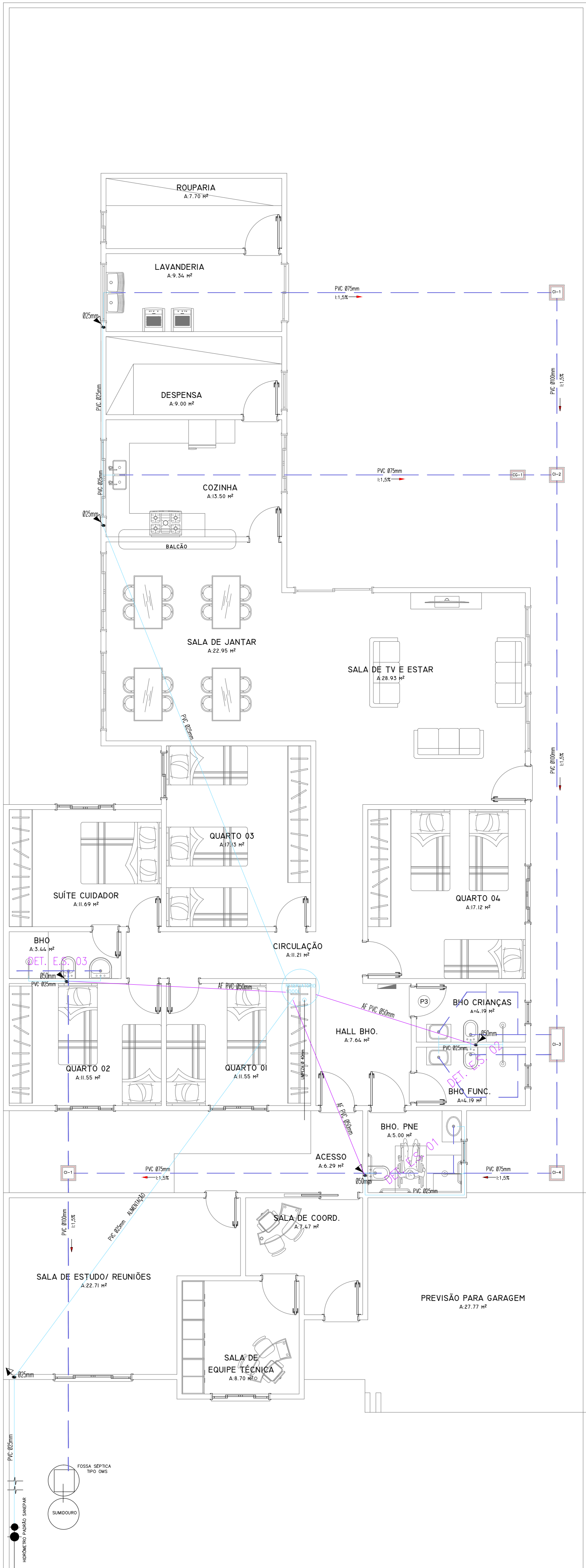
IMPLANTAÇÃO - ÁGUA FRIA E ESGOTO SANITÁRIO escala: 1/75
