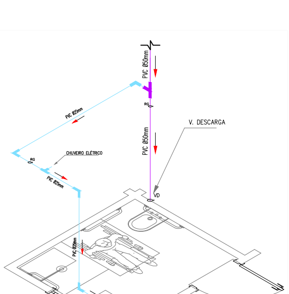
DET. ISOMÉTRICO ÁGUA FRIA 04 escala: 1/50
