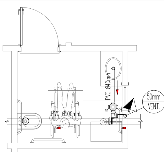
DET. ESGOTO SANITÁRIO 01 escala: 1/50
