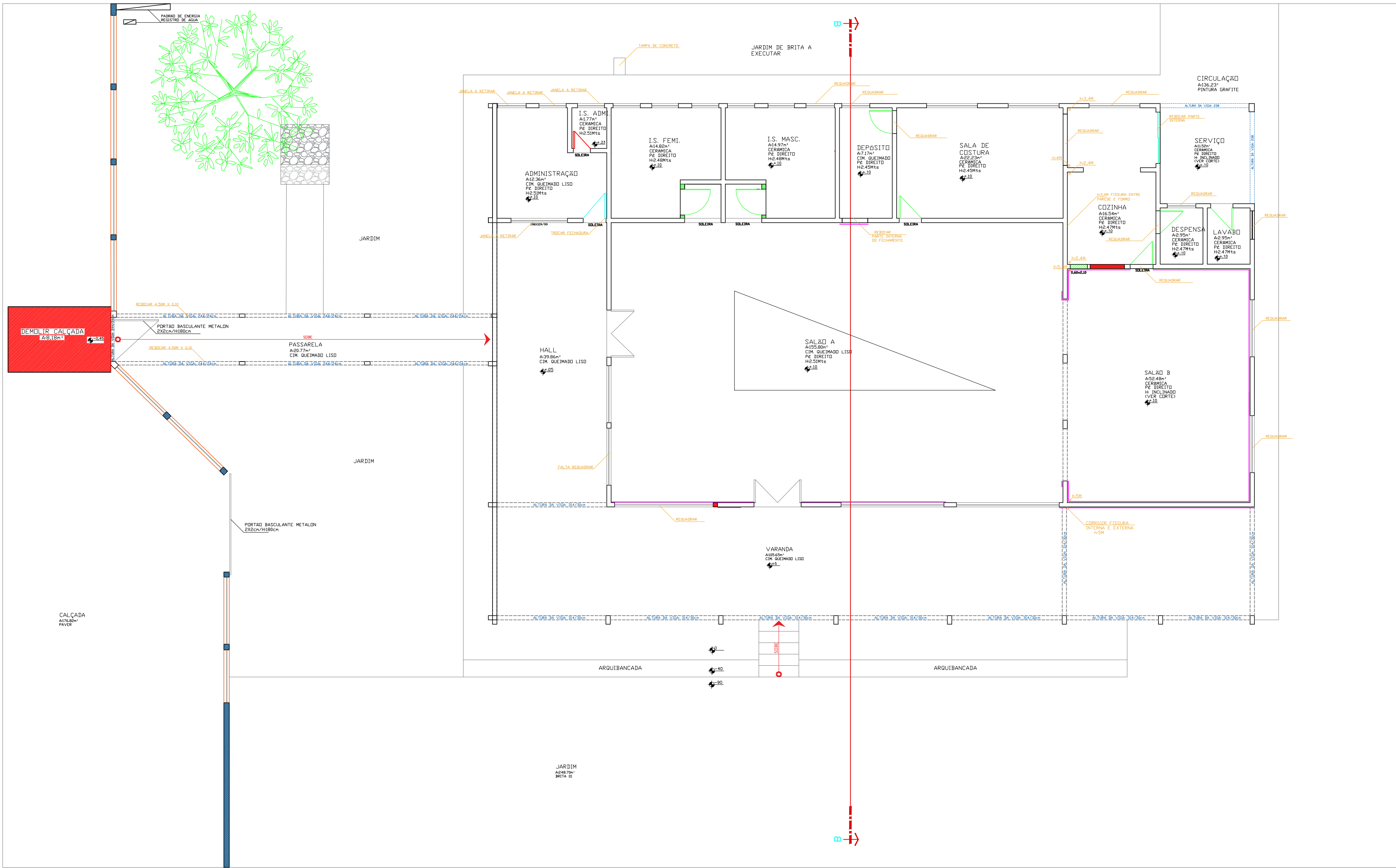
PLANTA BAIXA - CONSTRUIR/DEMOLIR Esc.: 1:100
