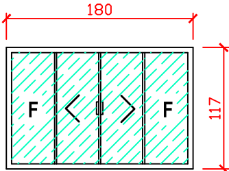
Det. J5 ESC. - 1/50
