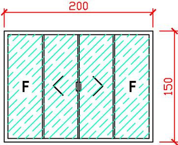
Det. J1 ESC. - 1/50
