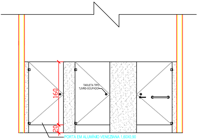
Vista A - I.S. Fem/Masc. ESC. - 1/50
