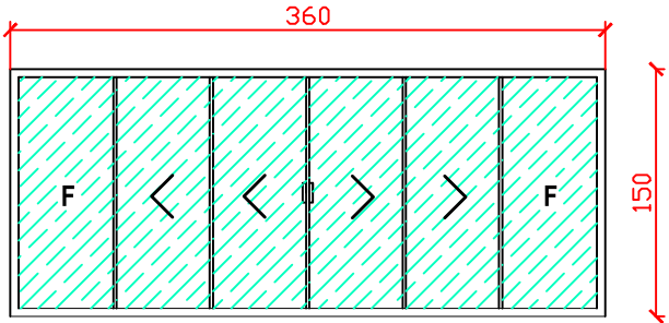
Det. J2 ESC. - 1/50
