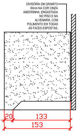
Det Divisória Granito ESC. - 1/50
