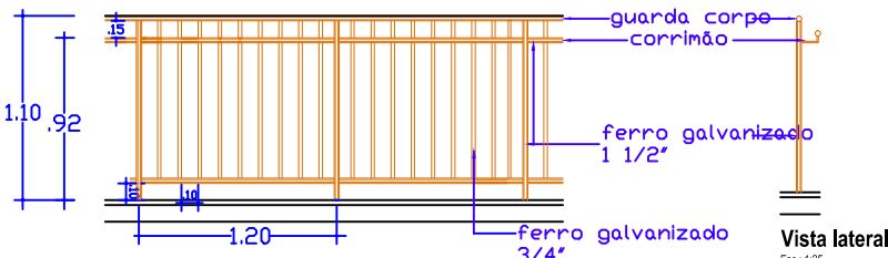
Det Guarda Corpo/ Corrimão ESC. - 1/50
