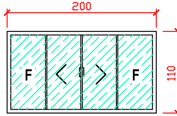
Det. J3 ESC. - 1/50
