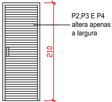
Det. P2, P3 E P4 ESC. - 1/50
