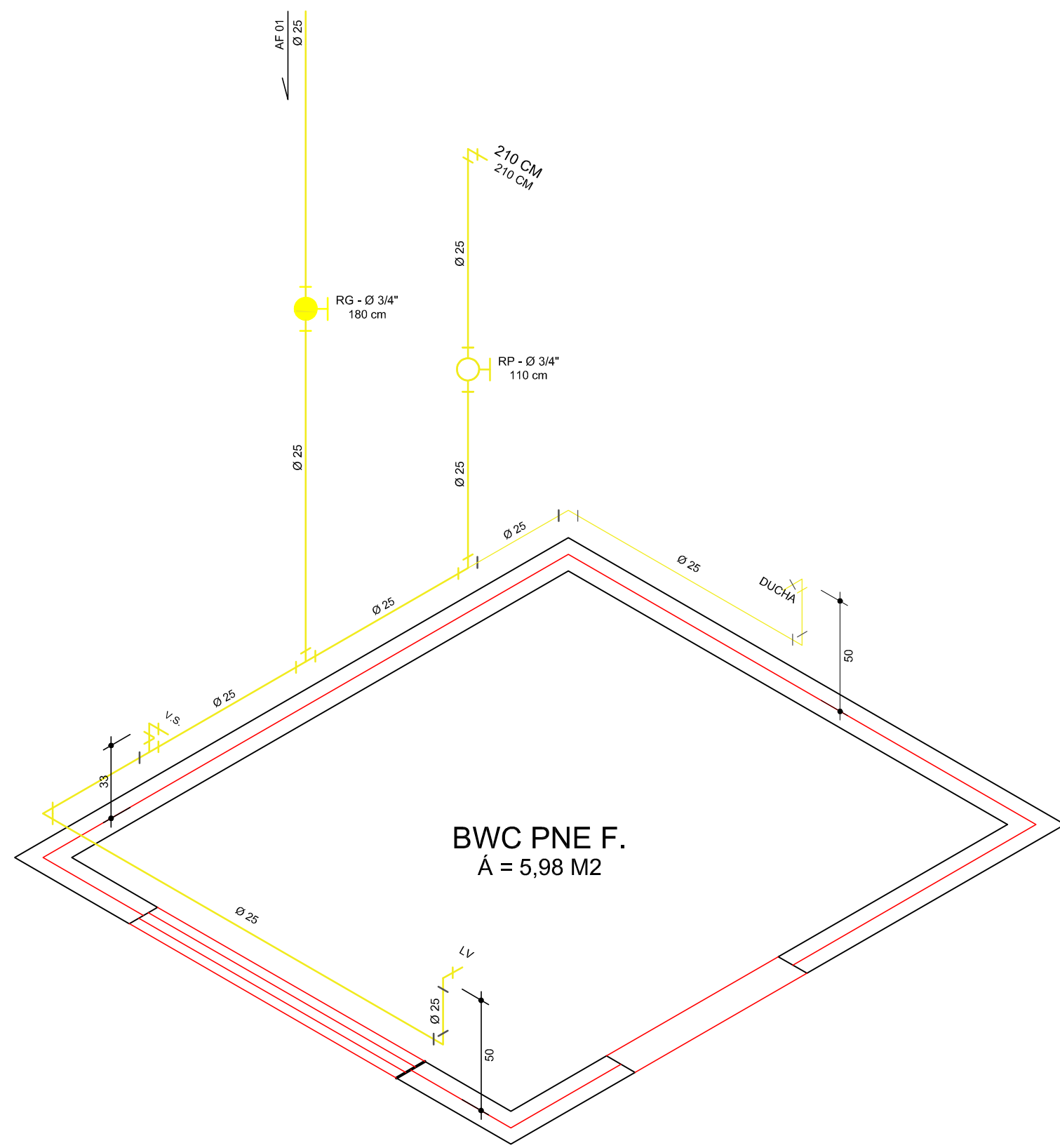
ISOMÉTRICO - 01 ESCALA 1 : 25
