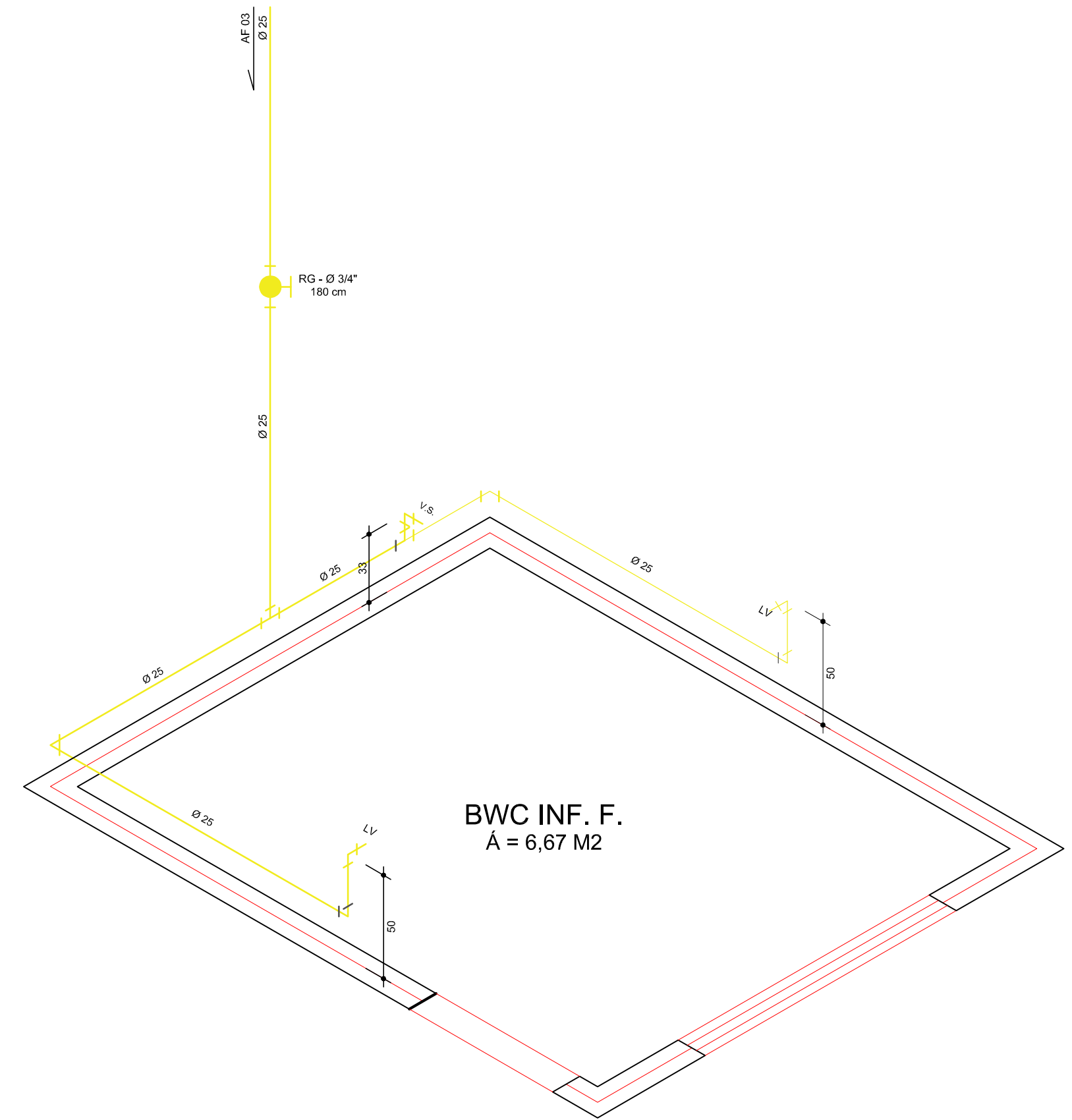
ISOMÉTRICO - 03 ESCALA 1 : 25
