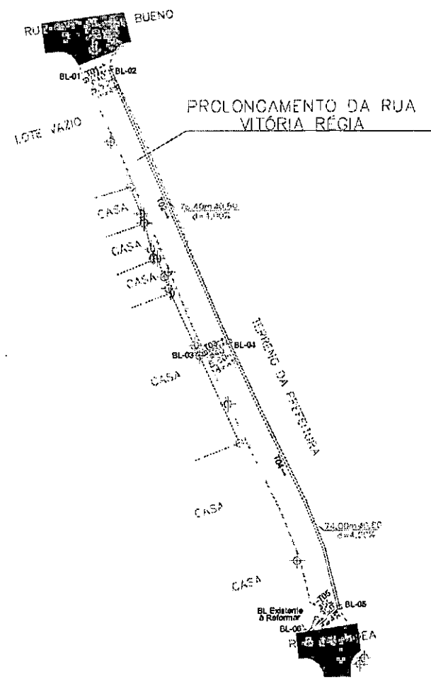
PLANTA DE DRENAGEM SEM ESCALA
