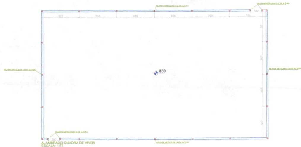
ALAMBRADO QUADRA DE AREIA ESCALA: 1:75
