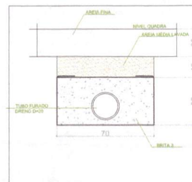
DRENO QUADRA DE AREIA ESCALA: 1:50
