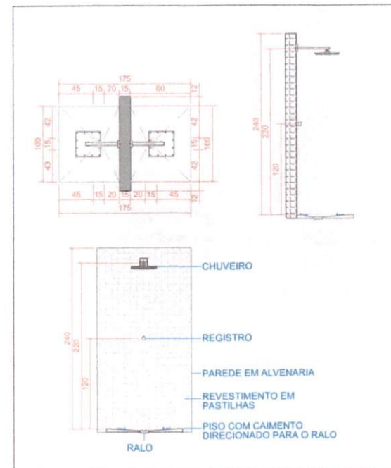
DETALHAMENTO DUCHAS ESCALA: 1:25
