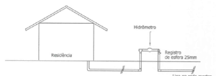
ESQUEMA DAS LIGAÇÕES DOMICILIARES
