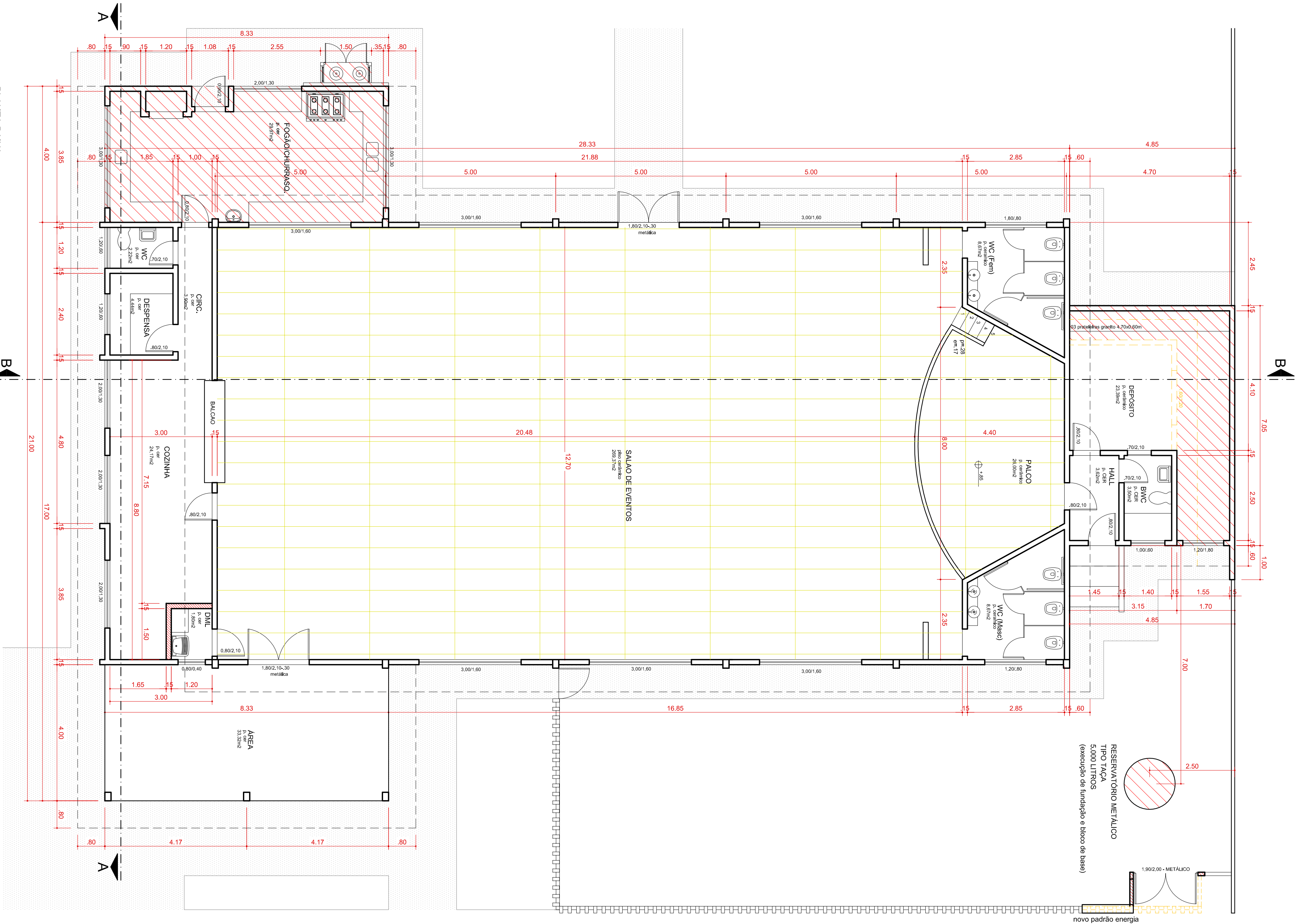
PLANTA BAXA ESQ.: 1:25
