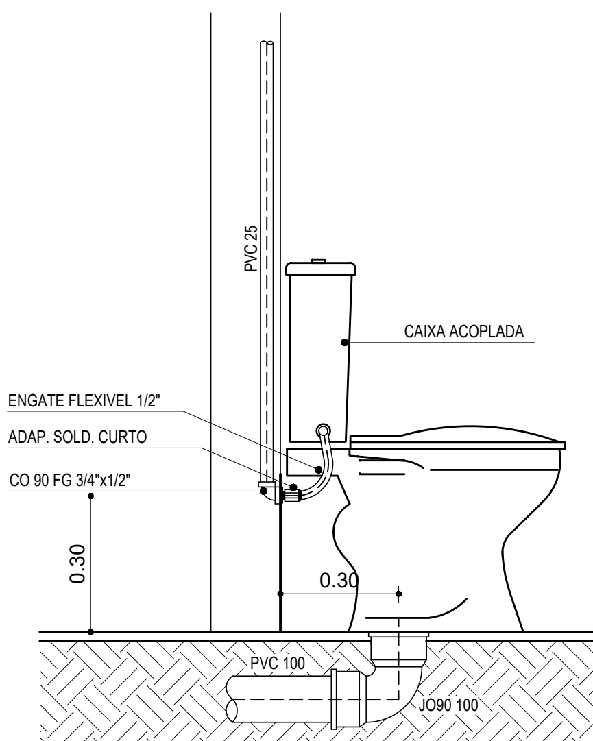
Det./ Vaso Sanitário c/ Caixa Acoplada S/ESCALA
