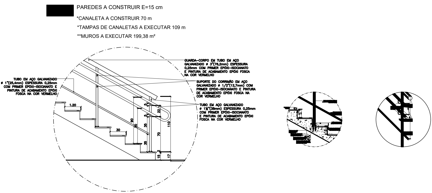
DETALHE GUARDA -CORPO RAMPAS E ESCADA SEM ESCALA
