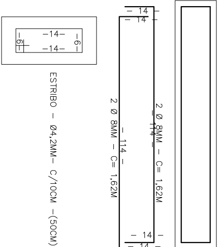
VIGA DE APOIO – GRADE (10X20)CM CONCRETO – FCK = 20 mpa.
