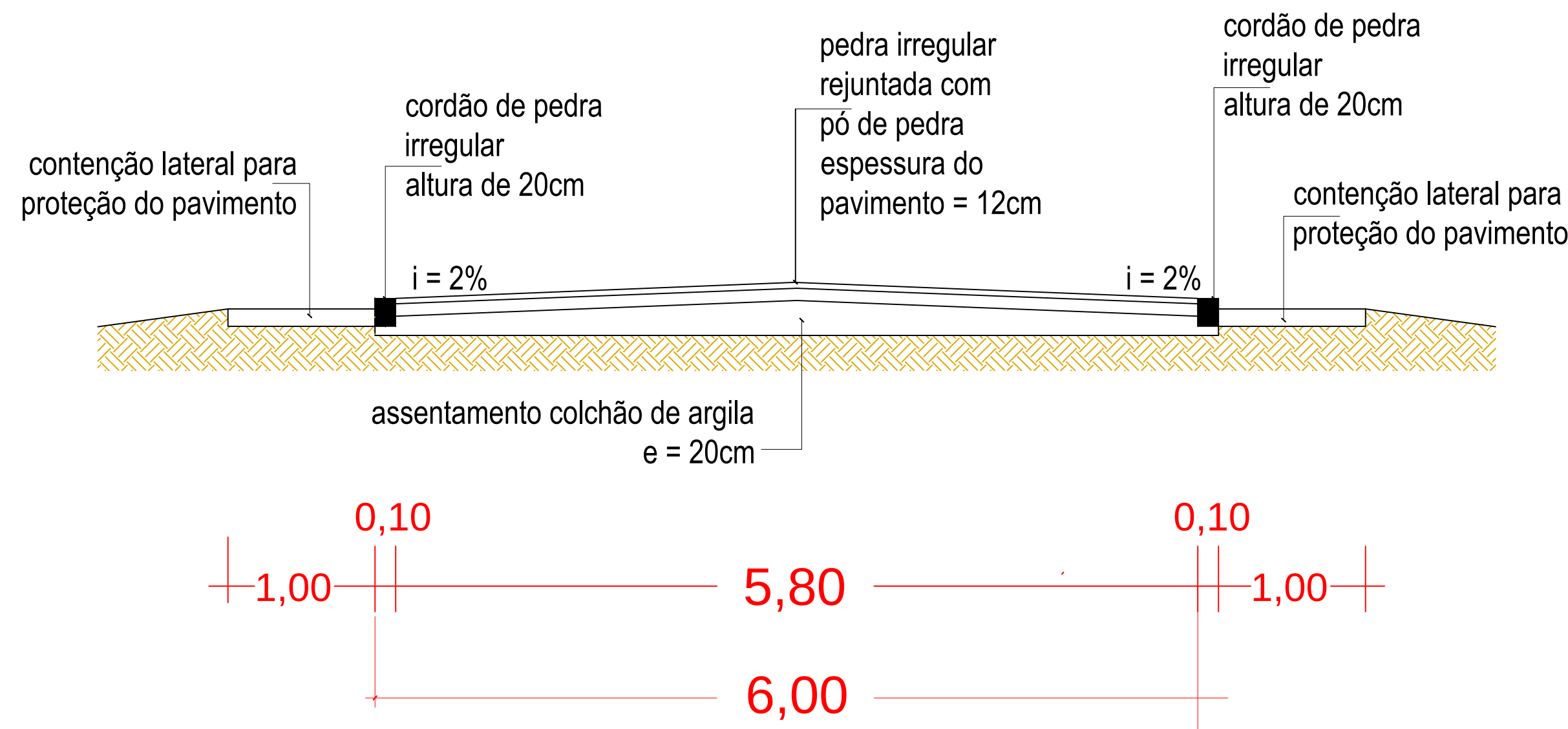
SEÇÃO TRANSVERSAL DA ESTRADA CORTE AA - Sem escala
