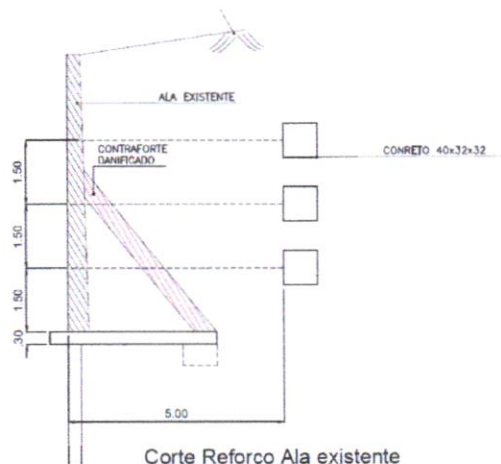
Corte Reforço Ala existente
