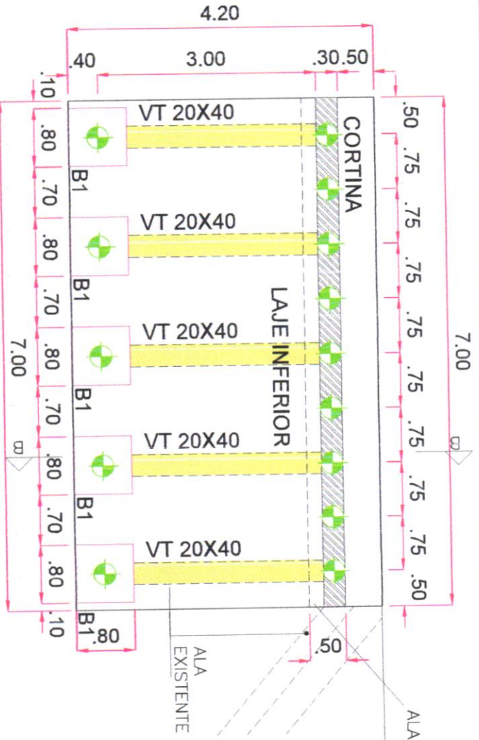
Forma Vigas e Cortina Escala 1:50
