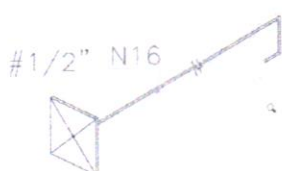
Detalhe Tirante de reforço - 15 unid 6m e 6 unid 5m
