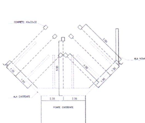
Detalhe Tirante de reforço - 15 unid 6m e 6 unid 5m
