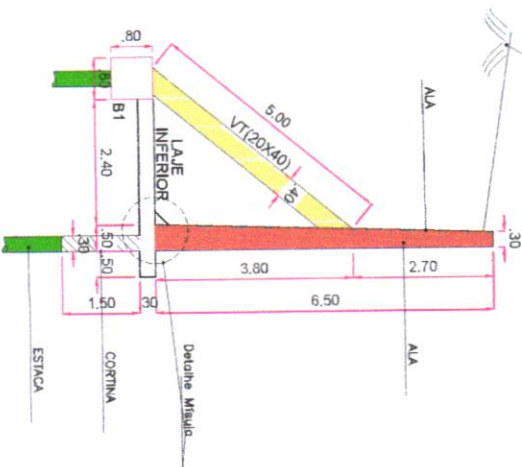
Forma - Corte B-B Escala 1:50
