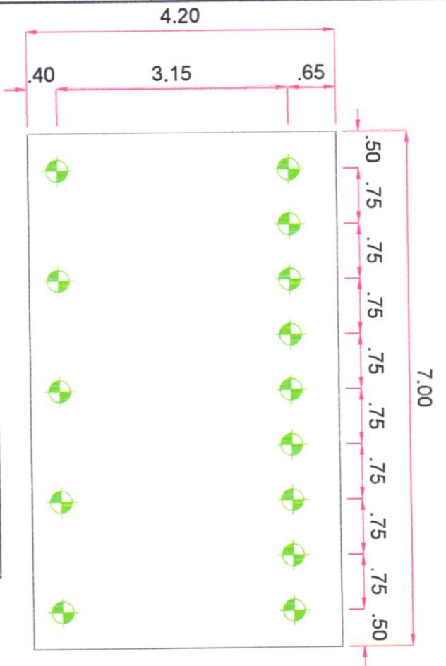
Locação das estacas Escala 1:50
