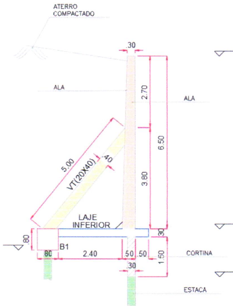
Corte Escala 1:50
