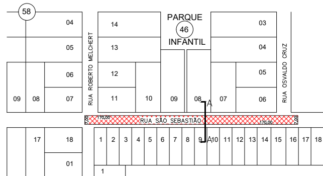
PLANTA Rua São Sebastião A=1.190,00 m 2 ESC. 1/100
