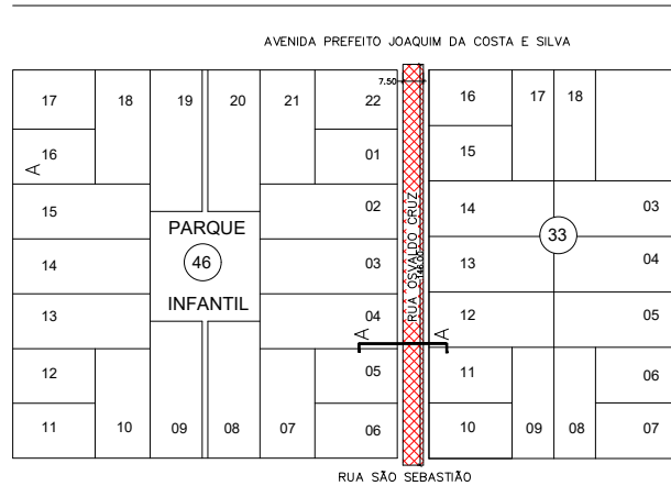
PLANTA Rua Osvaldo Cruz A=1.095,00 m 2 ESC. 1/100
