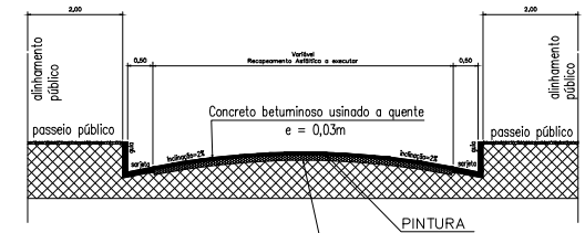
DET. DOS CORTES A-A - CBUQ s/ Esc.
