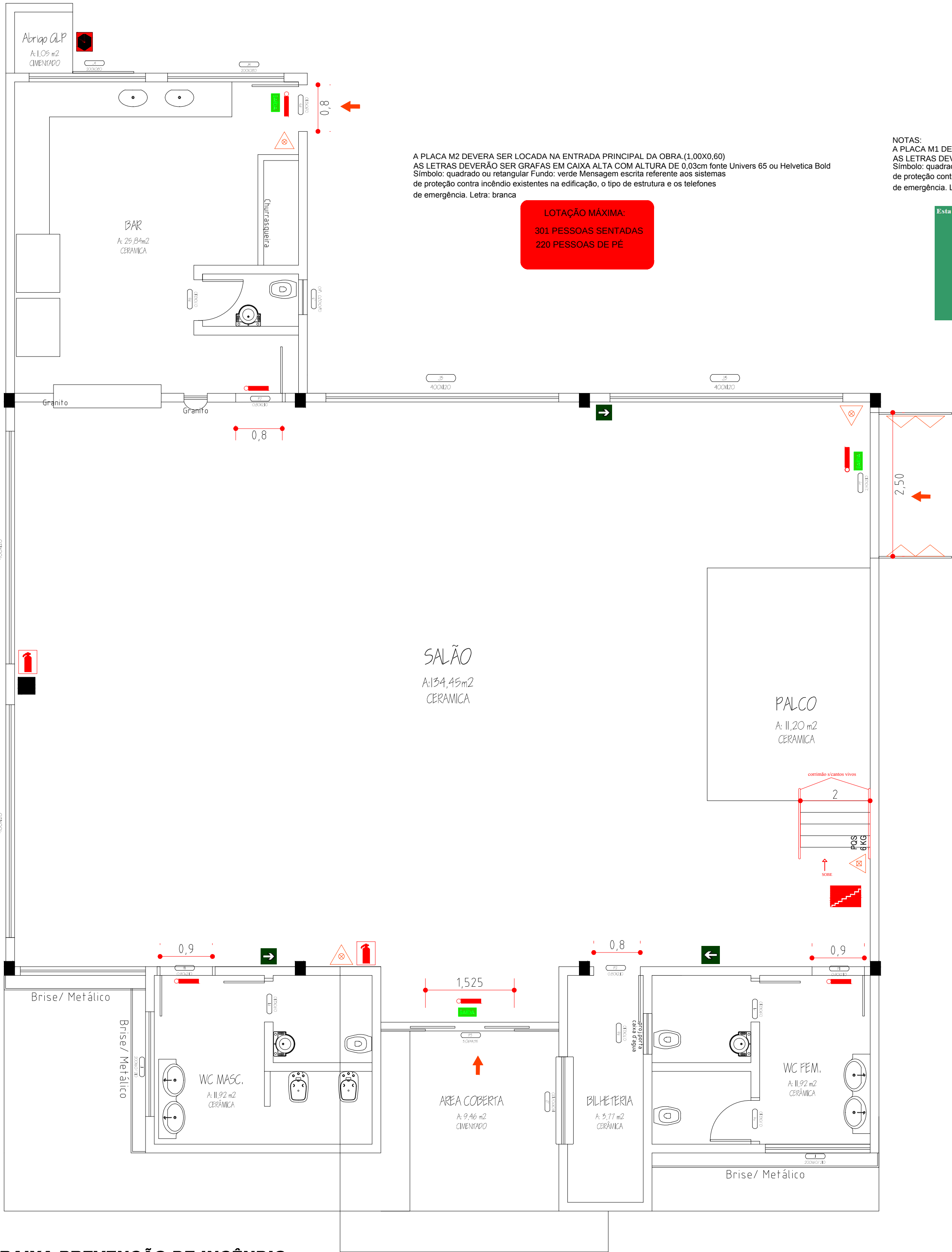
PLACA BAIXA-PREVENÇÃO DE INCÊNDIO ESCALA 1:50
