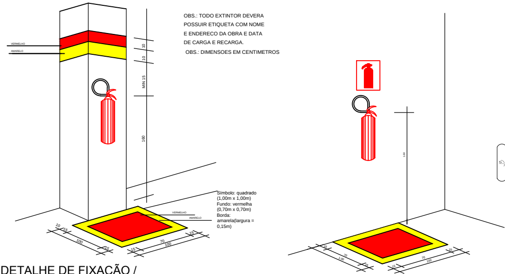
DETALHE DE FIXAÇÃO / SINALIZAÇÃO DOS EXTINTORES S/ ESCALA
