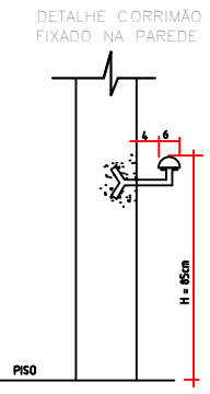
CORTE Sem escala
