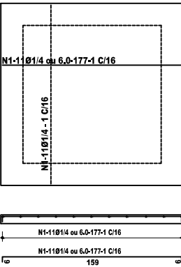
LAJE INFERIOR ESCALA 1/25
