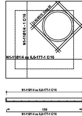
LAJE SUPERIOR ESCALA 1/25
