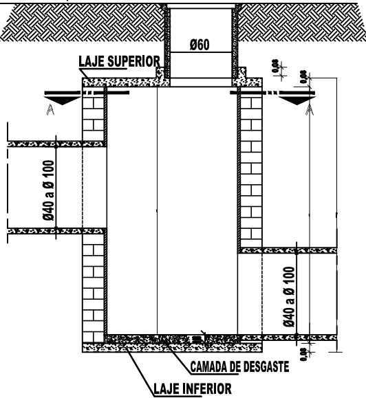
CORTE BB ESCALA 1/25
