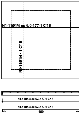
LAJE INFERIOR ESCALA 1/25
