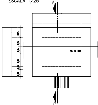
VISTA SUPERIOR ESCALA 1/25
