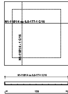
LAJE SUPERIOR ESCALA 1/25
