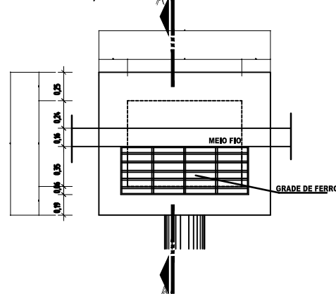
VISTA SUPERIOR ESCALA 1/25
