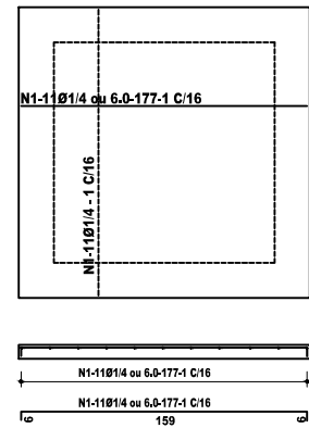
LAJE INFERIOR ESCALA 1/25
