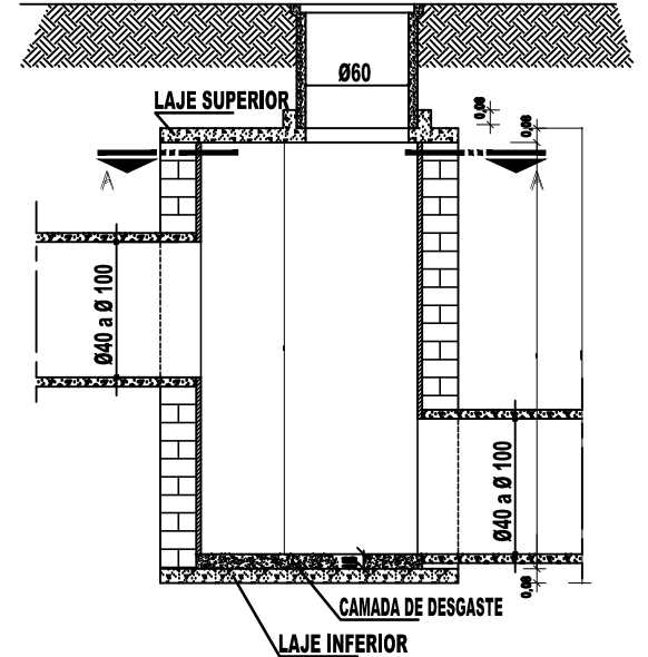
CORTE BB ESCALA 1/25
