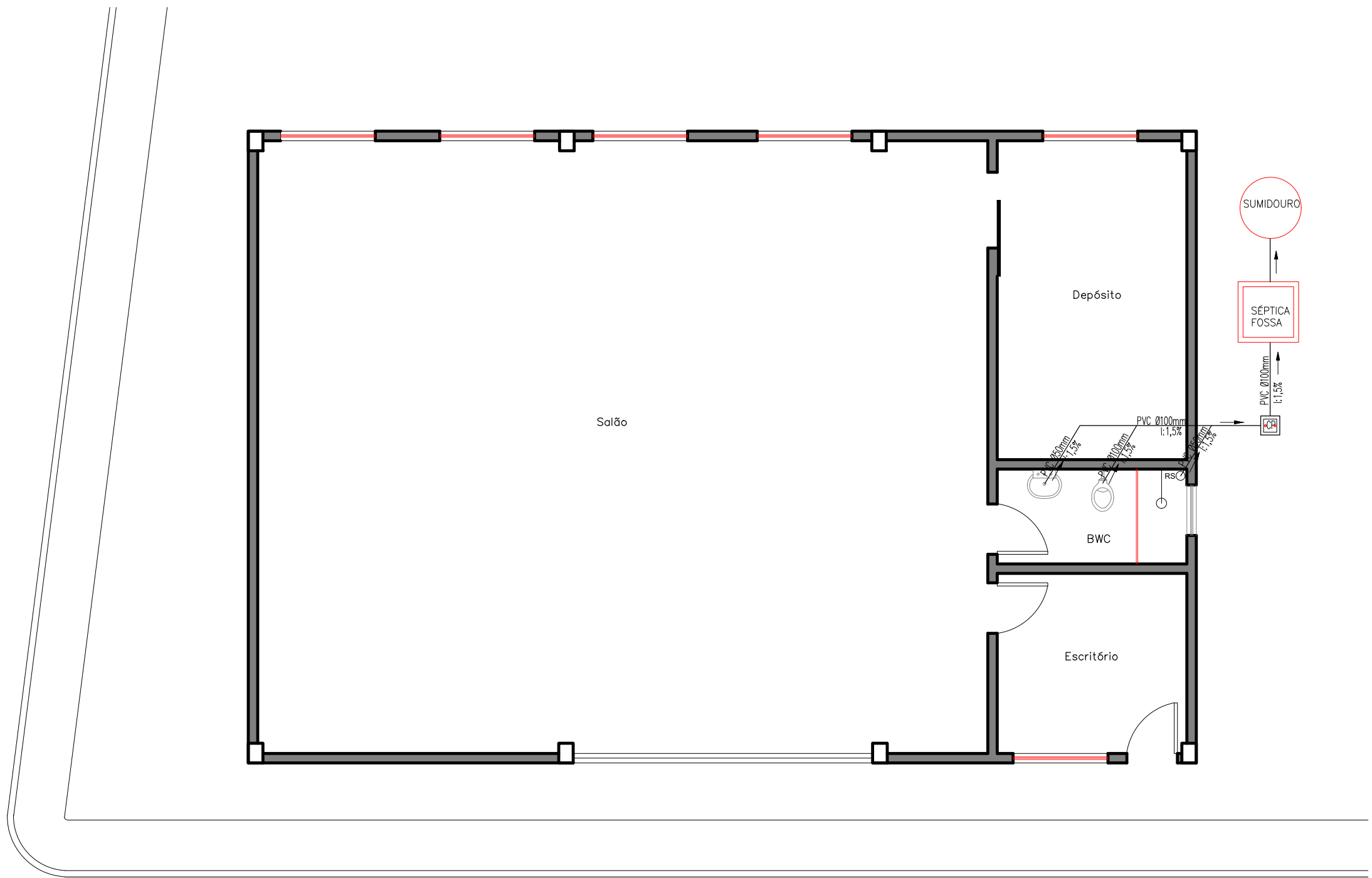
PLANTA BAIXA - ESGOTO SANITÁRIO ESC.1/75
