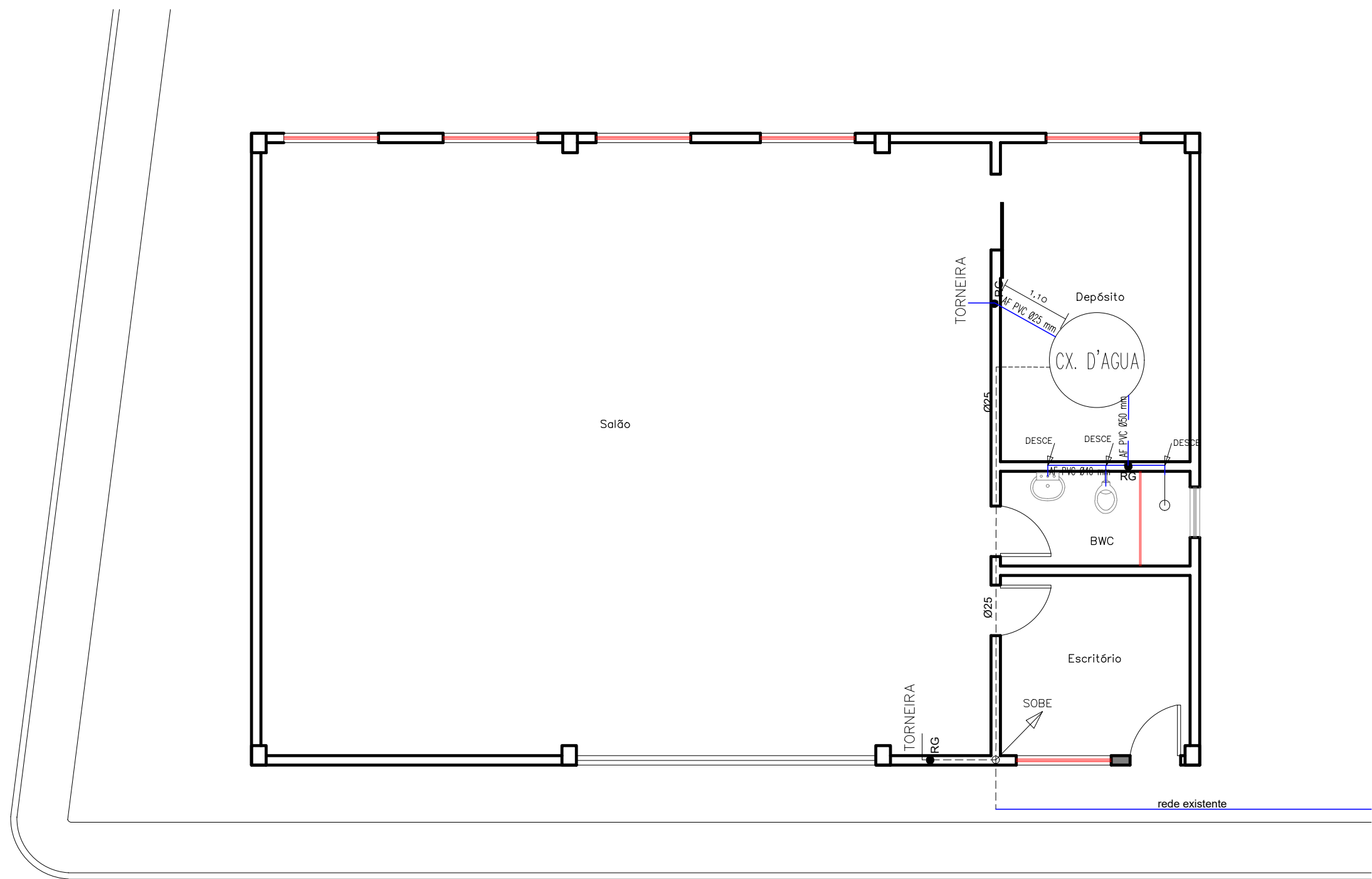
PLANTA BAIXA - ÁGUA FRIA ESC.1/75
