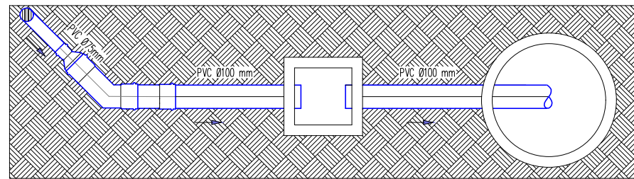
DETALHE DE LIGAÇÃO ESGOTO ESCALA 1:20
