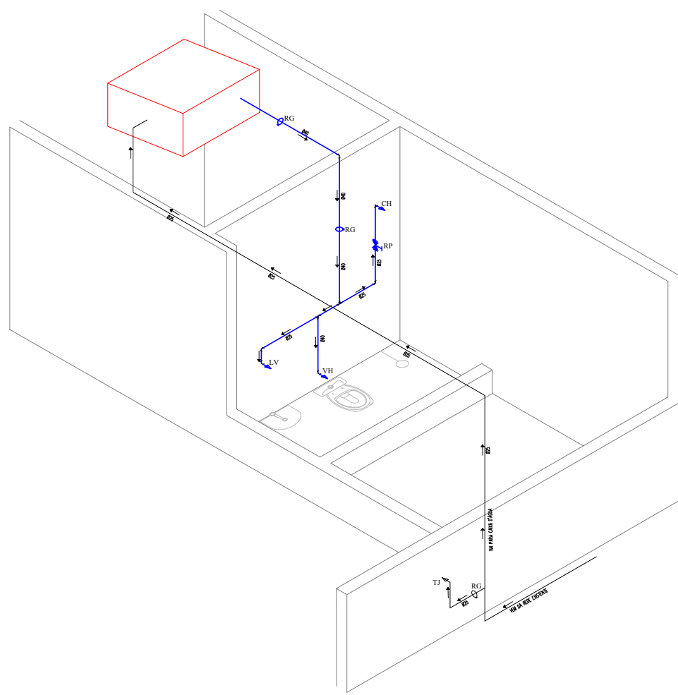
DET. ISOMÉTRICO ÁGUA FRIA ESCALA 1:100
