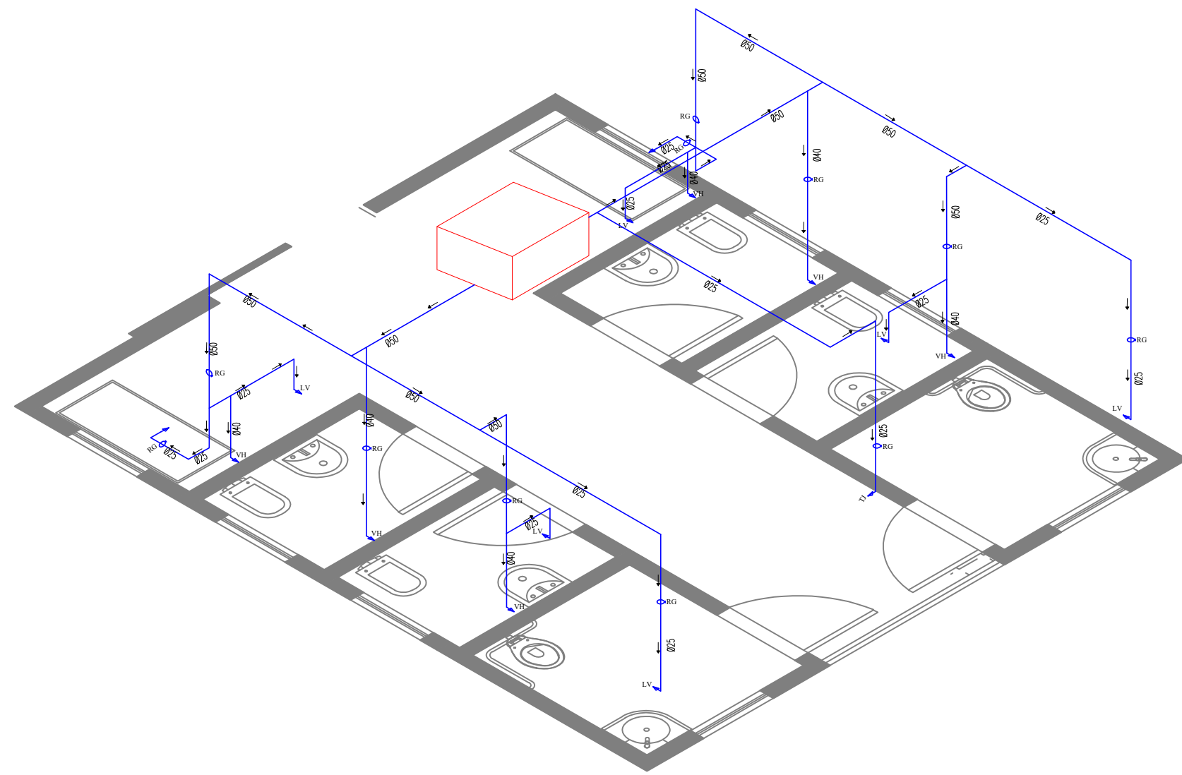
DET. ISOMÉTRICO ÁGUA FRIA ESCALA 1:100
