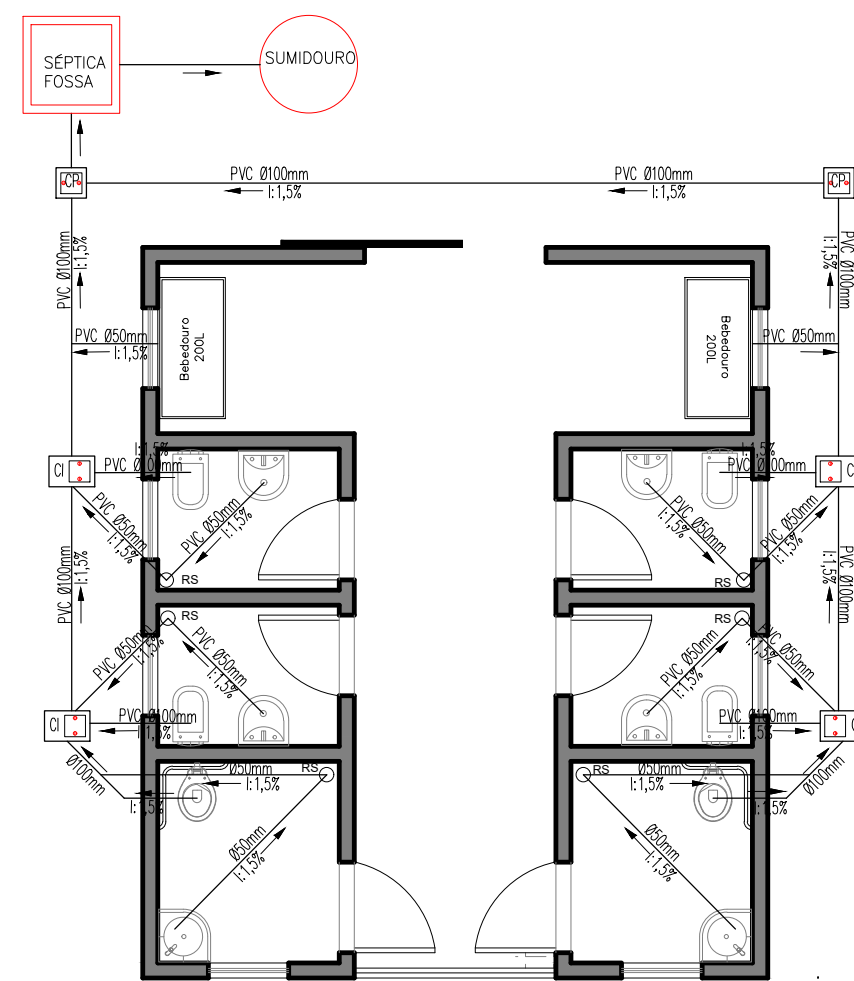
PLANTA BAIXA - ESGOTO SANITÁRIO ESC.1/75
