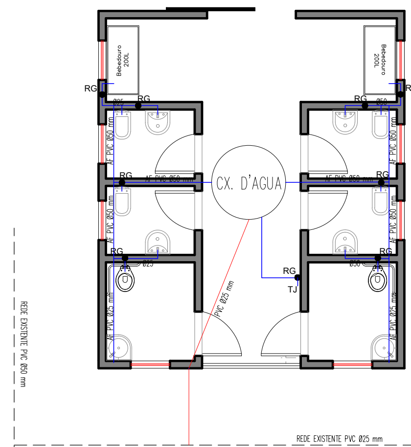
PLANTA BAIXA - ÁGUA FRIA ESC.1/75
