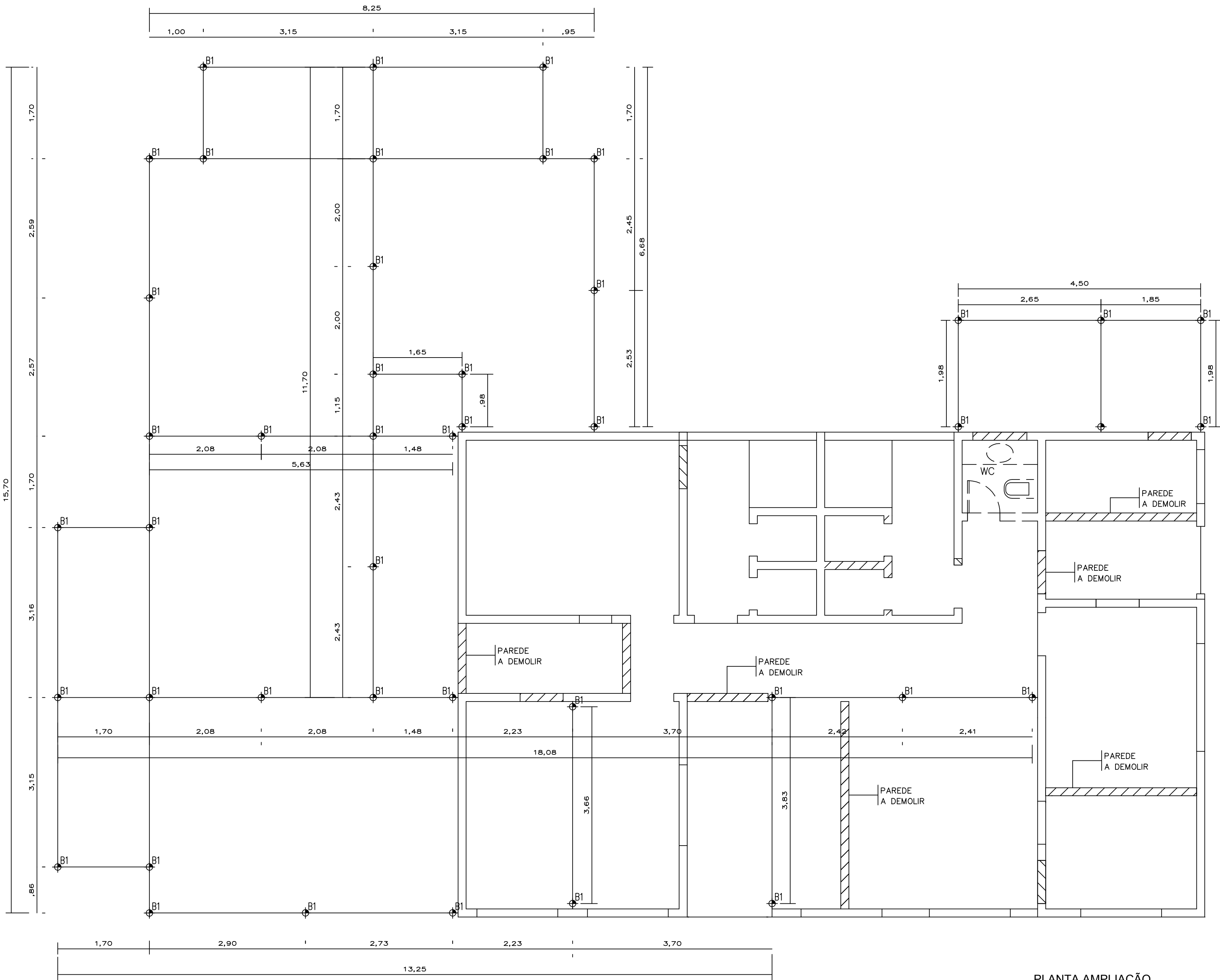
PLANTA AMPLIAÇÃO Escala 1/50
