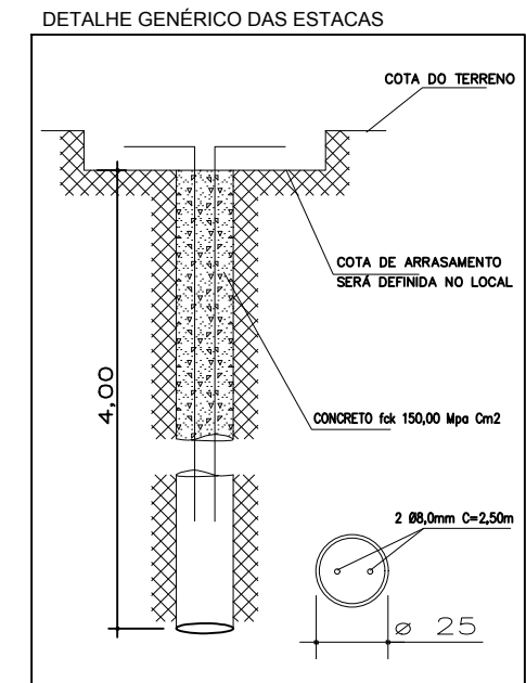
ESTACA Ø 25Cm x 4,00m x 44
