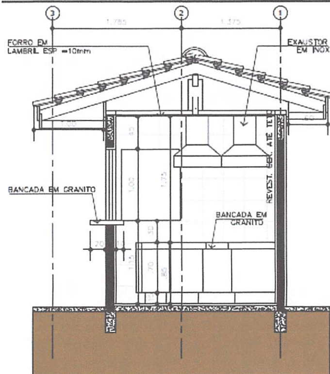
ELEVACÃO E1
