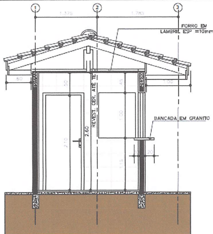
ELEVAÇÃO E3
