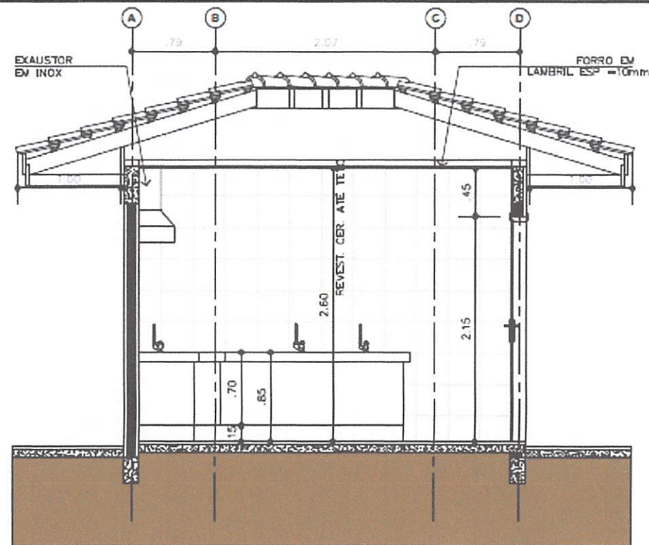
ELEVACÃO E2
