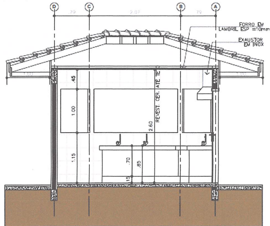
ELEVAÇÃO E4
