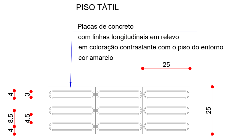
DETALHES DO PISO TÁTIL DIRECIONAL - 2951 unidades PLANTA ESCALA 1:10
