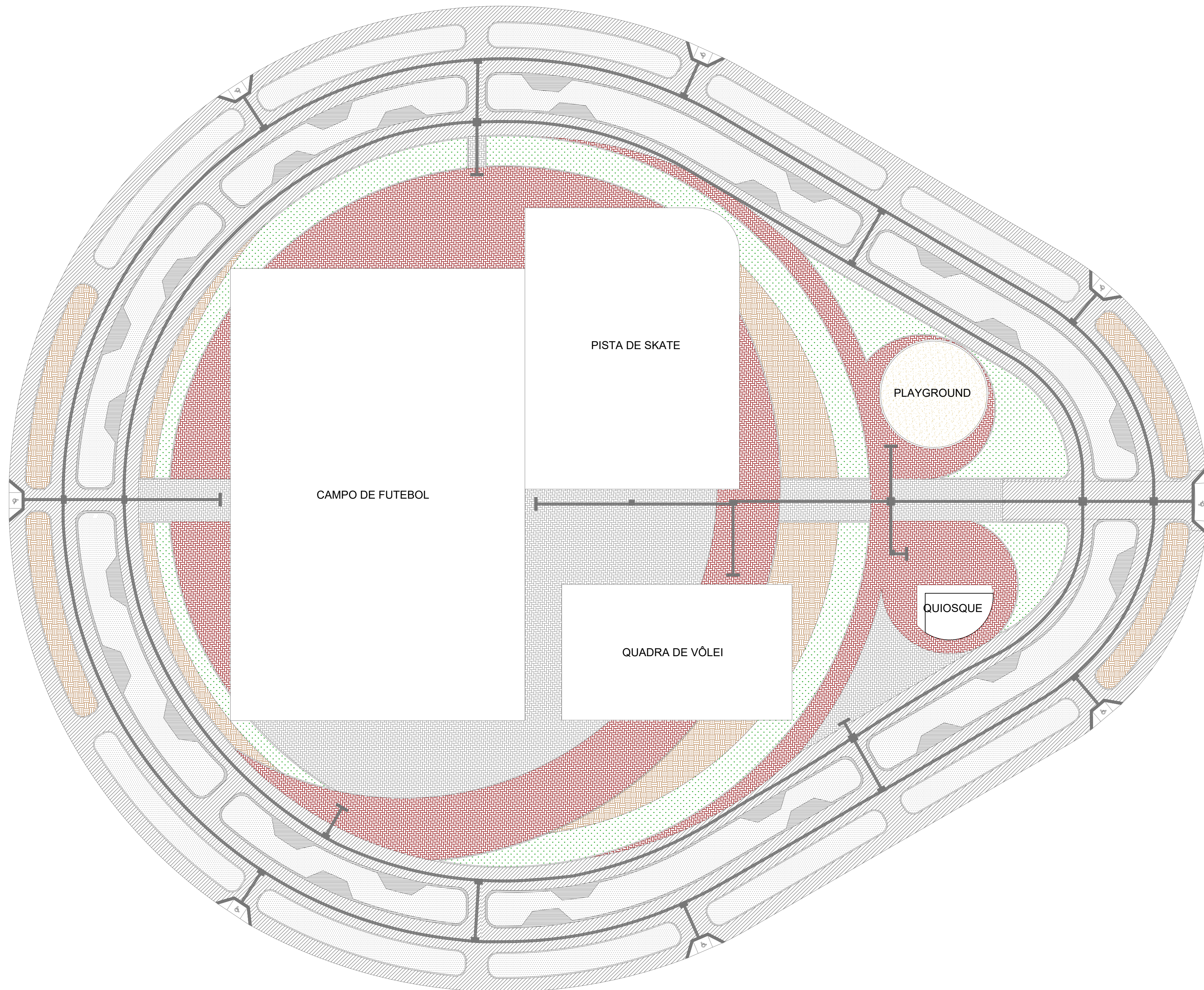
PLANTA DE PAGINAÇÃO E ROTAS ACESSÍVEIS PARA PNE ESCALA 1:250
