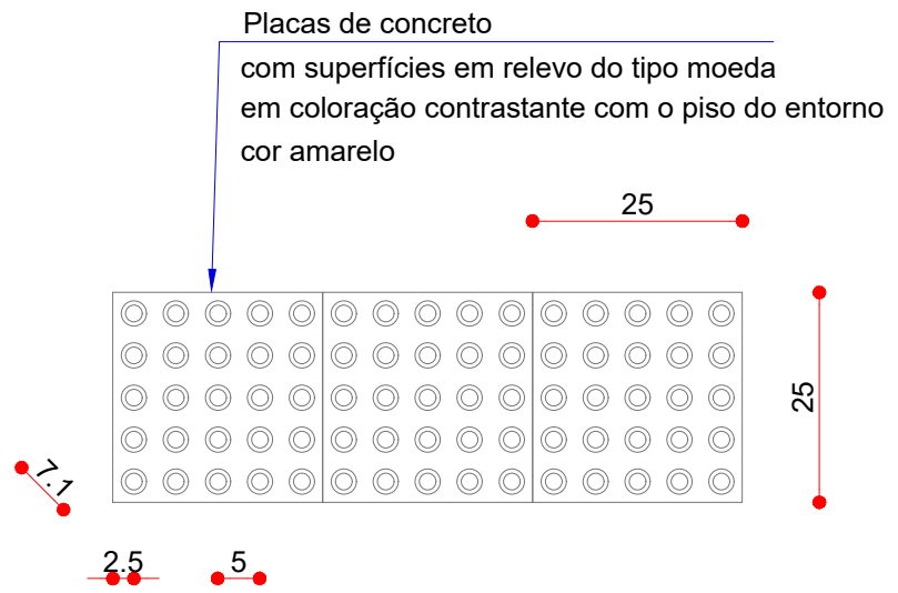
DETALHES DO PISO TÁTIL ALERTA - 413 unidades PLANTA ESCALA 1:10
