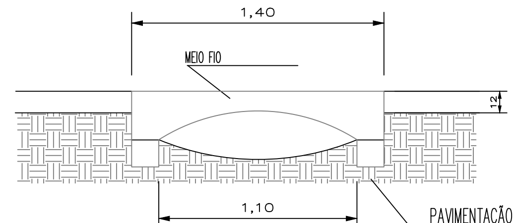
DETALHE BOCA DE LOBO
