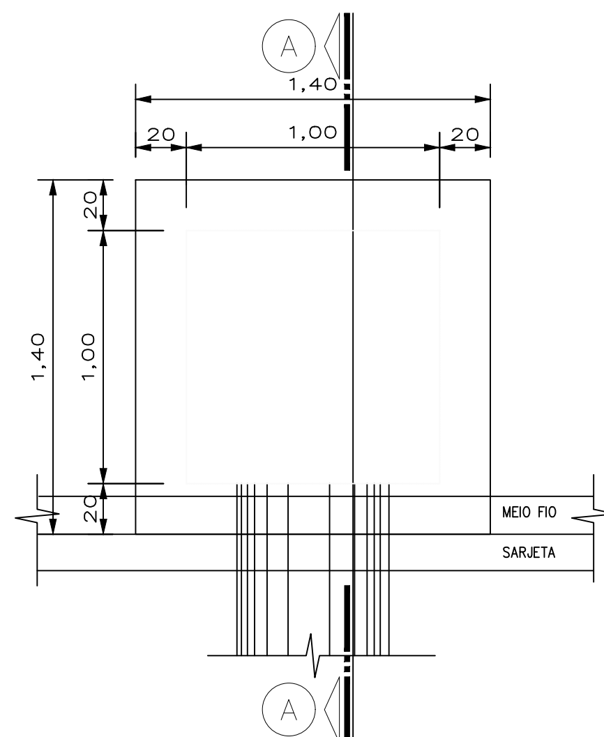
DETALHE BOCA DE LOBO VISTA SUPERIOR
