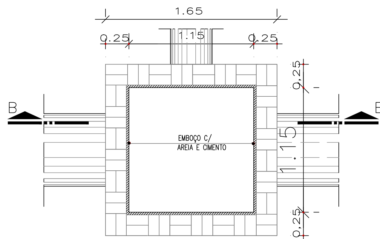
CAIXA DE LIGAÇÃO EM ALVENARIA CORTE AA
