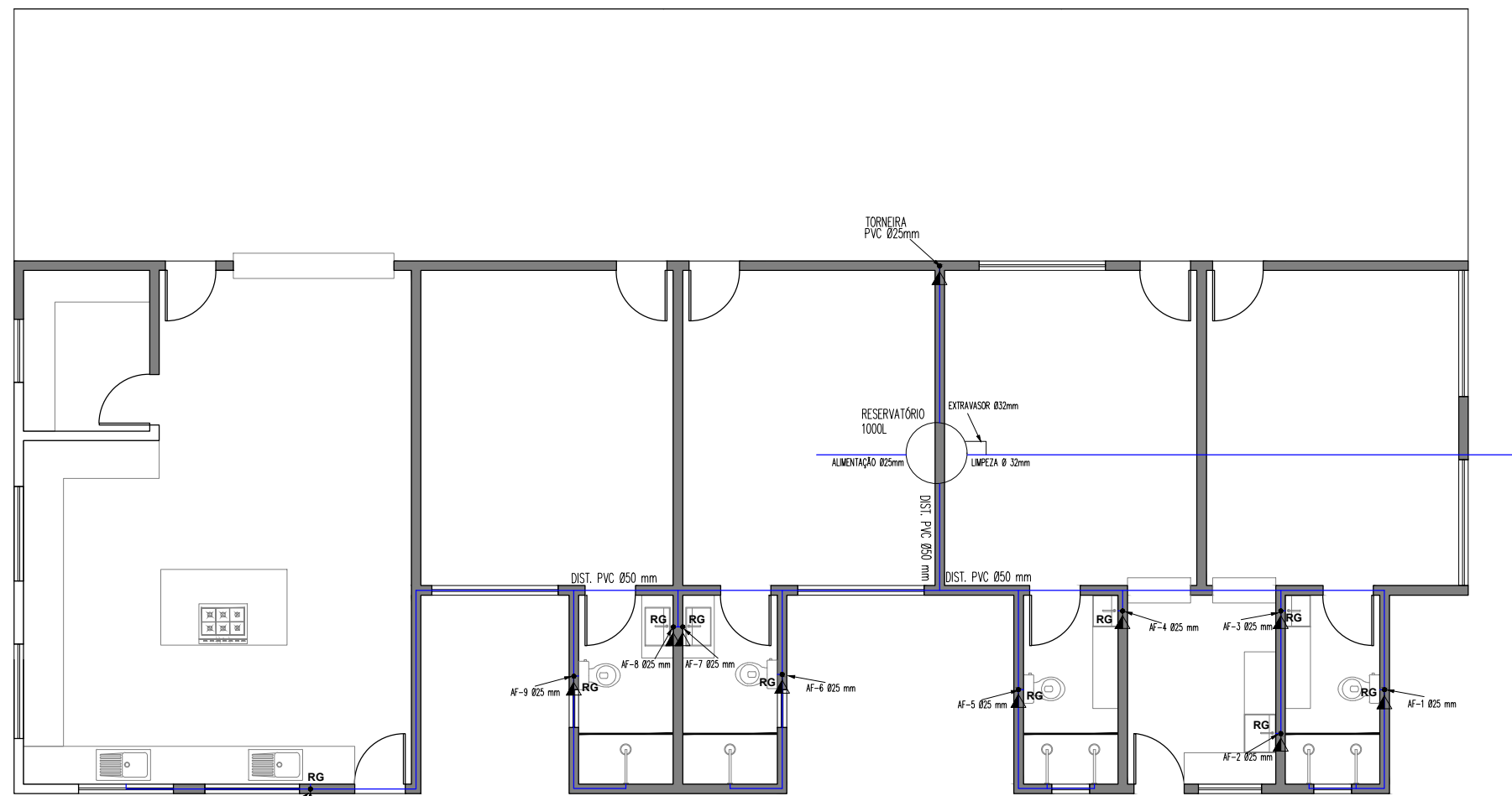
PLANTA BAIXA HIDRÁULICA — ESCALA 1:100
