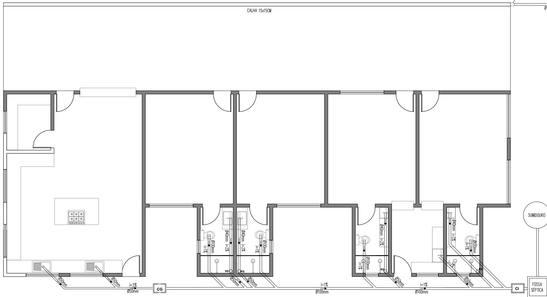
PLANTA BAIXA SANITÁRIA — ESCALA 1:100
