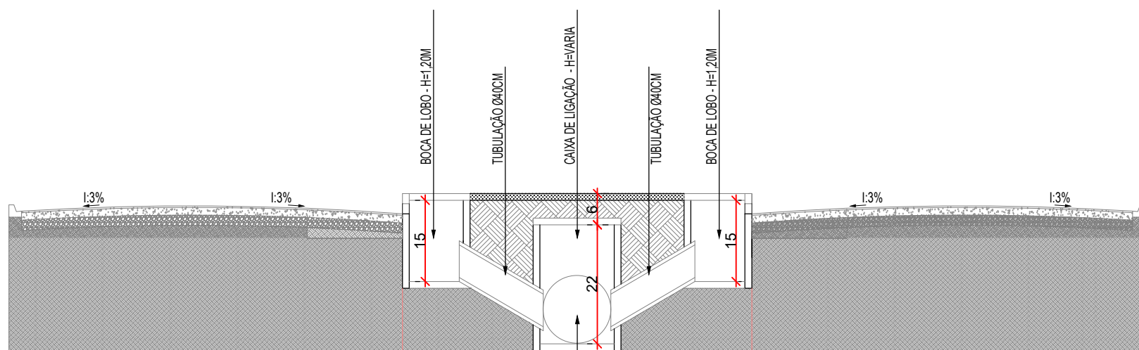
SEÇÃO TRANSVERSAL - DRENAGEM SEM ESC.
