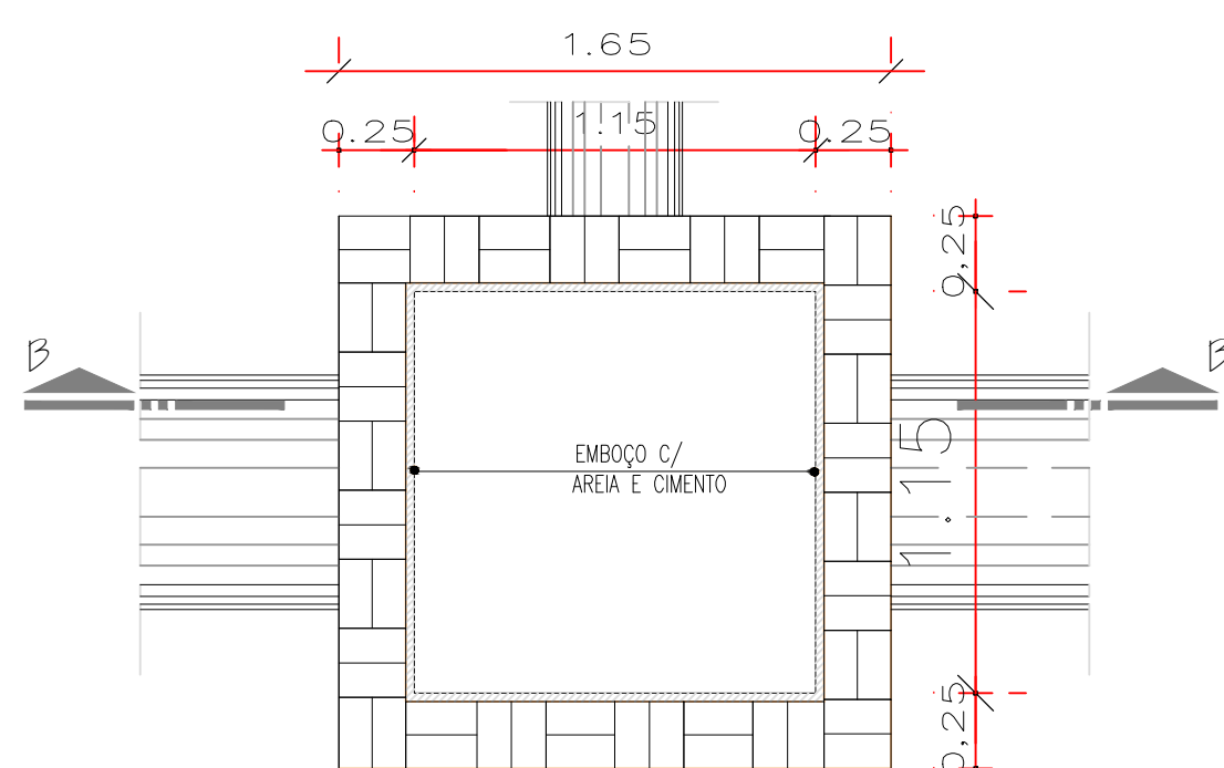
CAIXA DE LIGAÇÃO EM ALVENARIA CORTE AA
