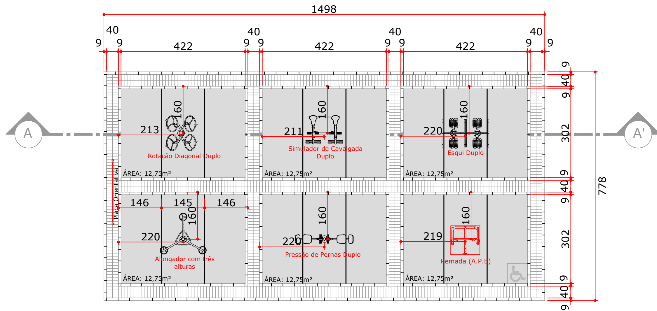
ATI - 04 esc.:1/100
