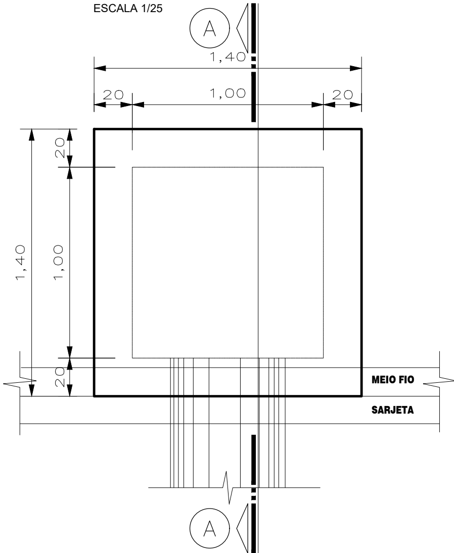
DETALHE BOCA DE LOBO VISTA SUPERIOR ESCALA 1/25
