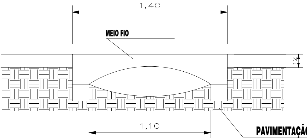
DETALHE DO MEIO-FIO ESCALA 1/12,5
