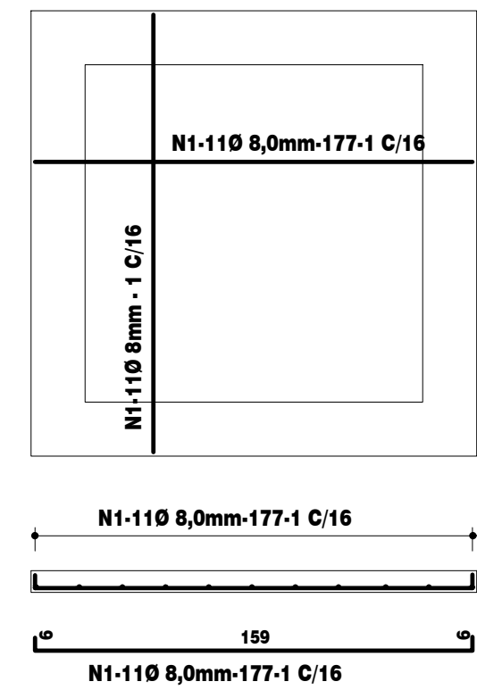
LAJE SUPERIOR ESCALA 1/25
