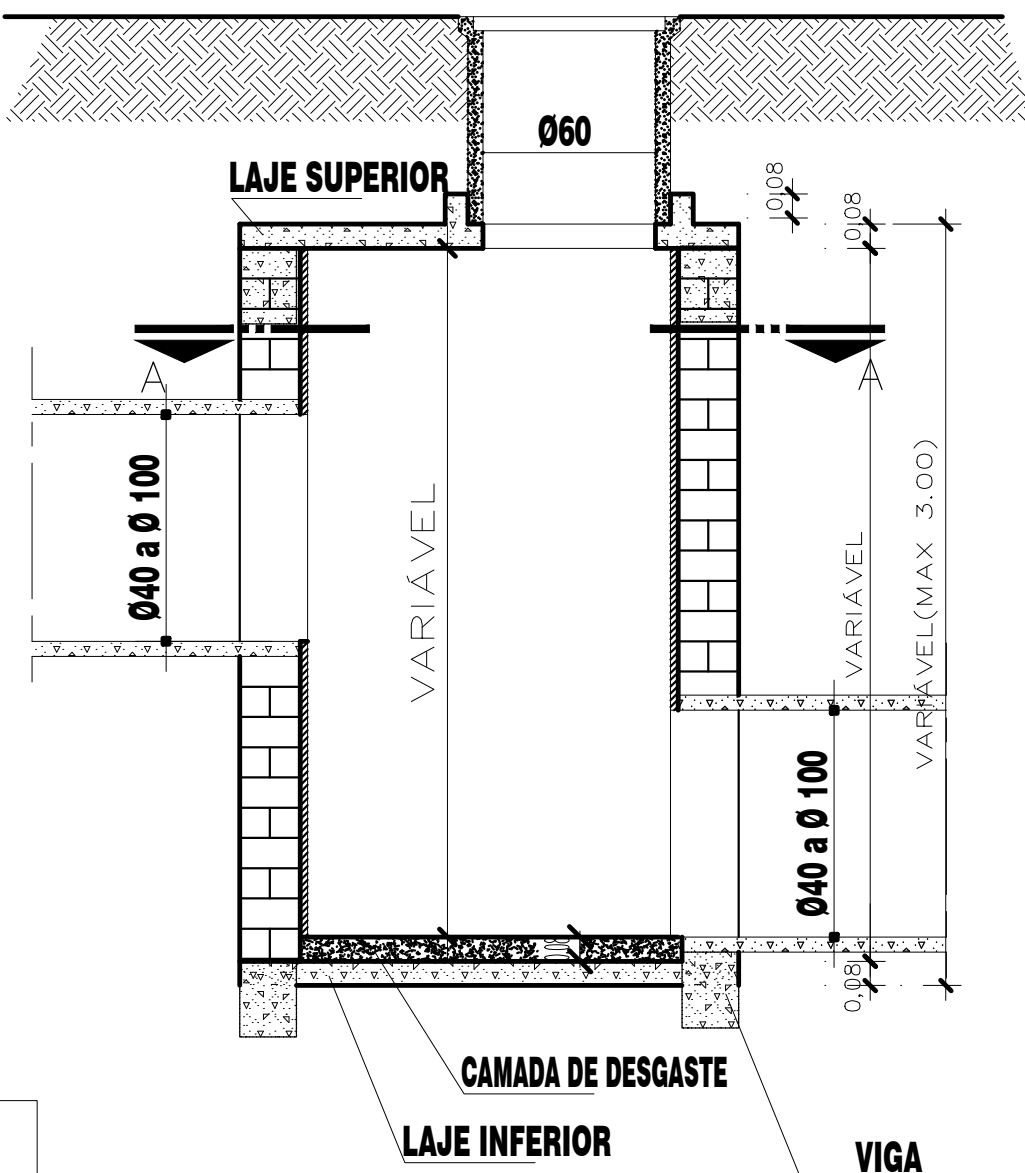
CORTE BB ESCALA 1/25
