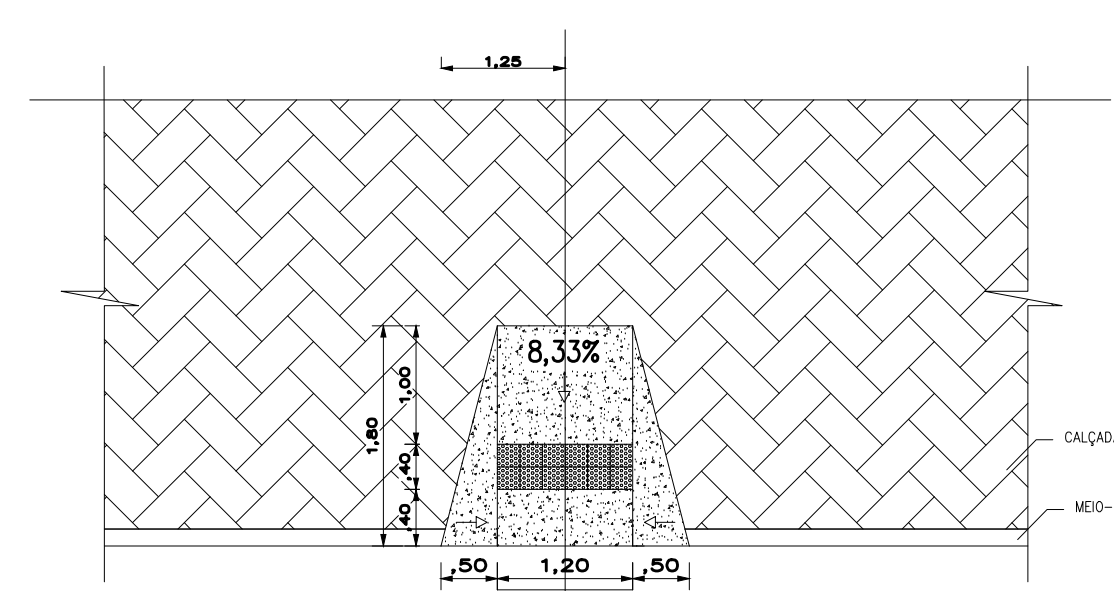
DETALHE DA RAMPA CALÇADA DE PAVER
