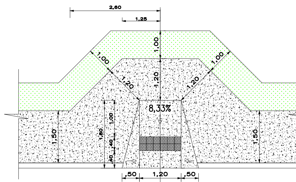
DETALHE DA RAMPA CALÇADA DE CONCRETO
