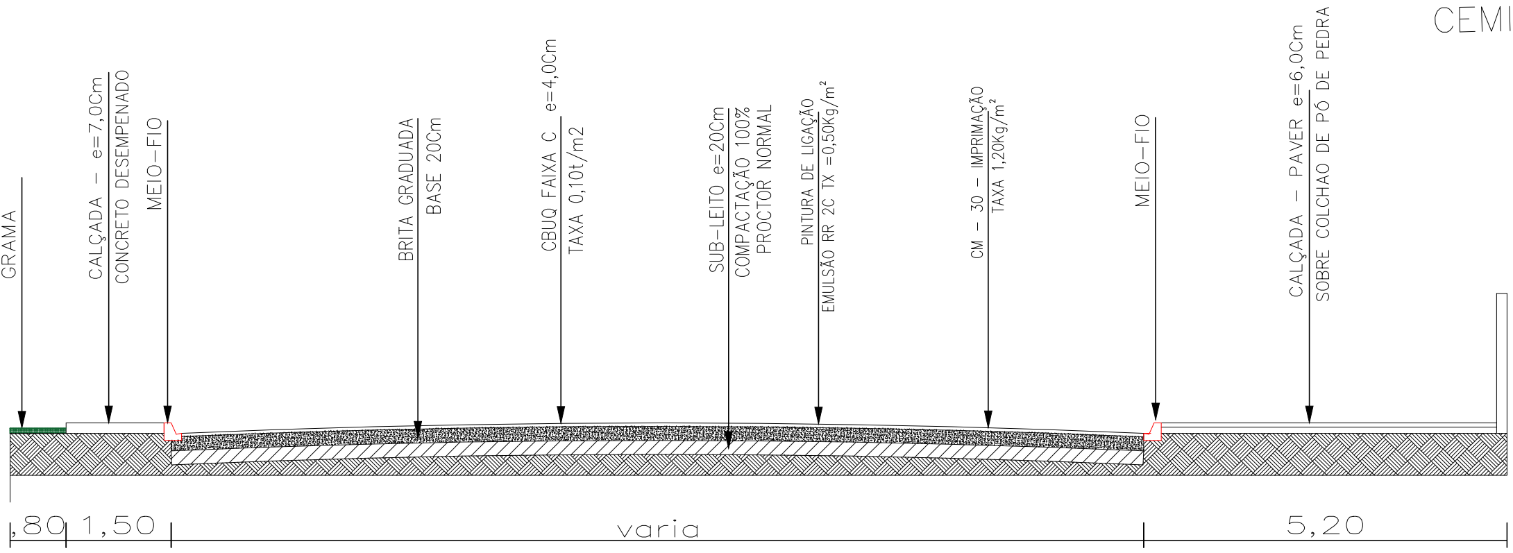
PERFIL TRANSVERSAL DA PISTA
