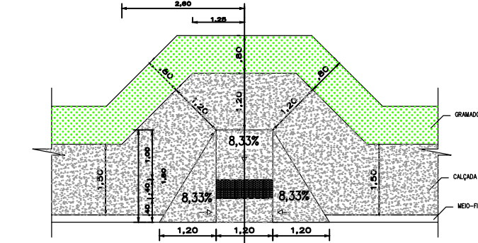
RUA DET. DO REBAIXO NA CALÇADA ESC. 1/50
