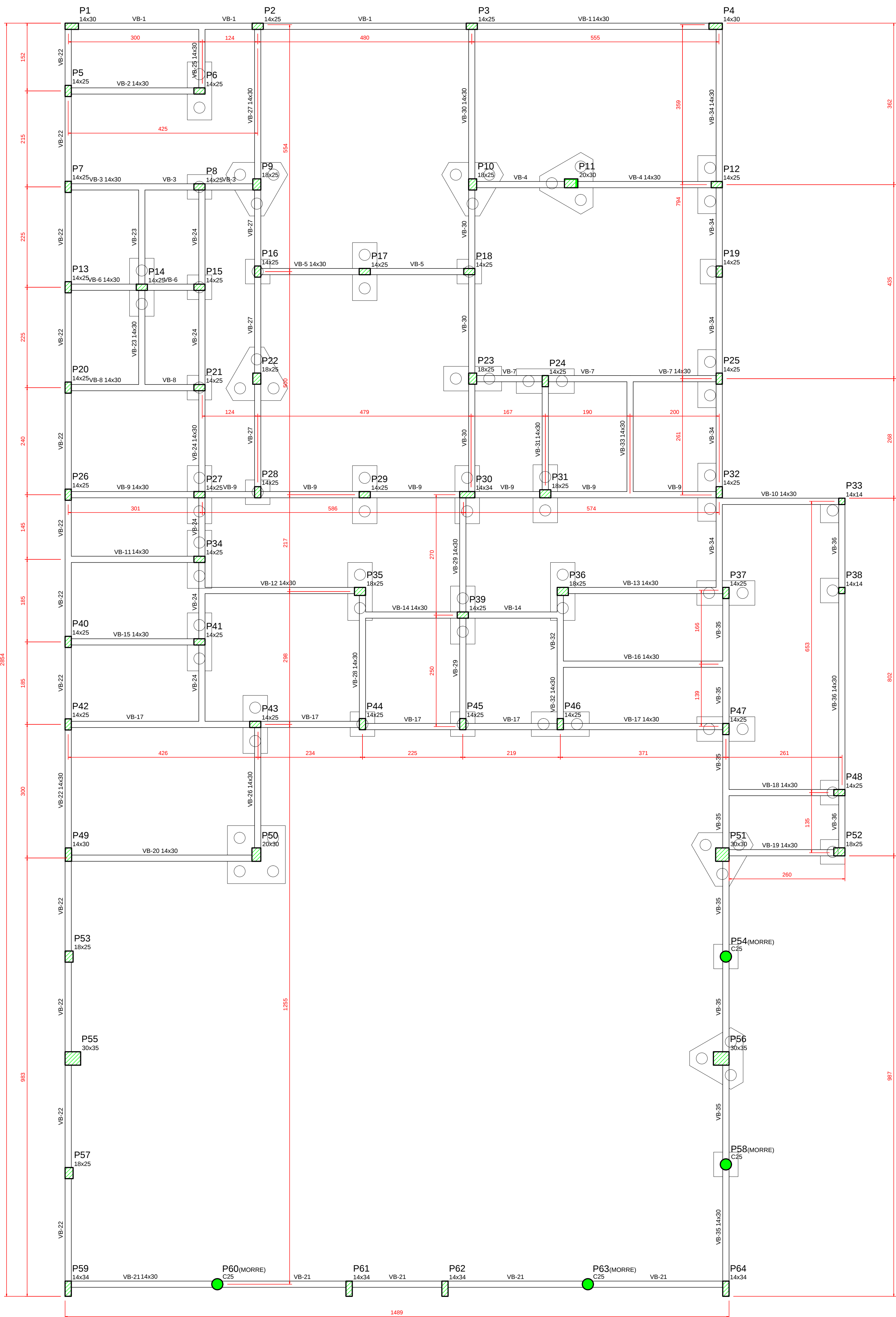
FORMA DAS VIGAS BALDRAME (-1,15) E (0,00)
