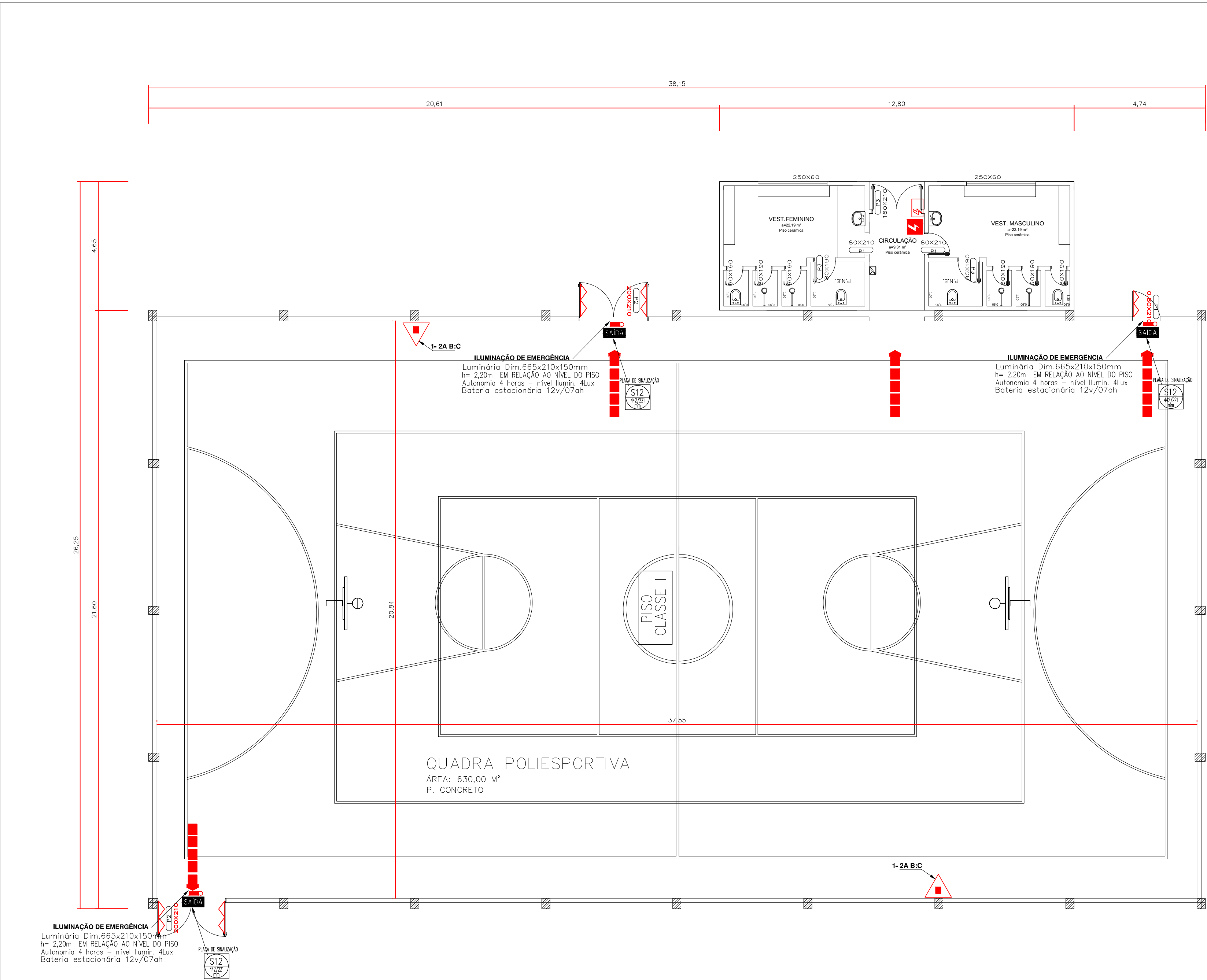
PLANTA BAIXA QUADRA POLIESPORTIVA Escala:1/100
