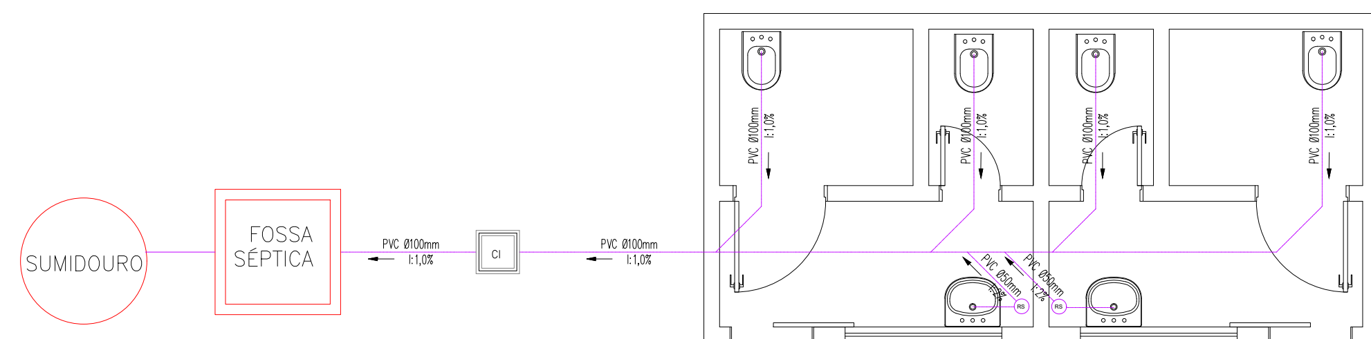
PLANTA BAIXA SANITÁRIA Escala 1/50
