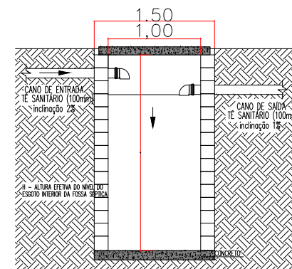
CORTE AA esc: 1/40
