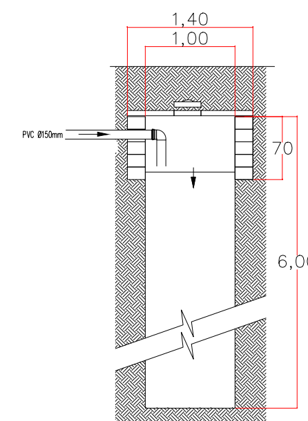
CORTE AA esc: 1/40
