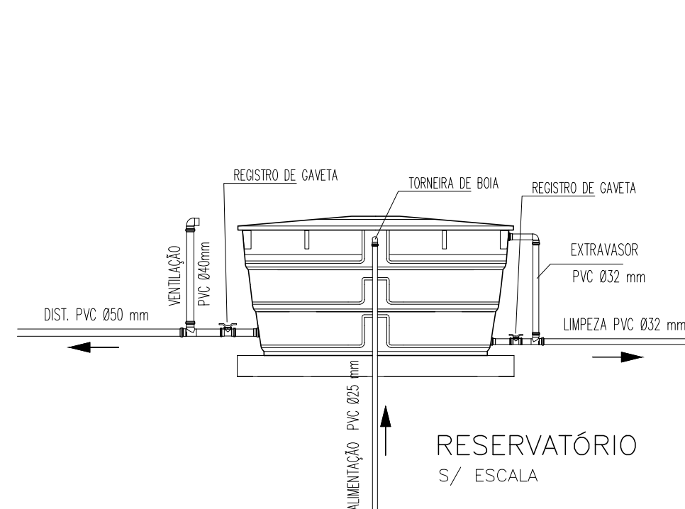
PLANTA BAIXA HIDRÁULICA Escala 1/50
