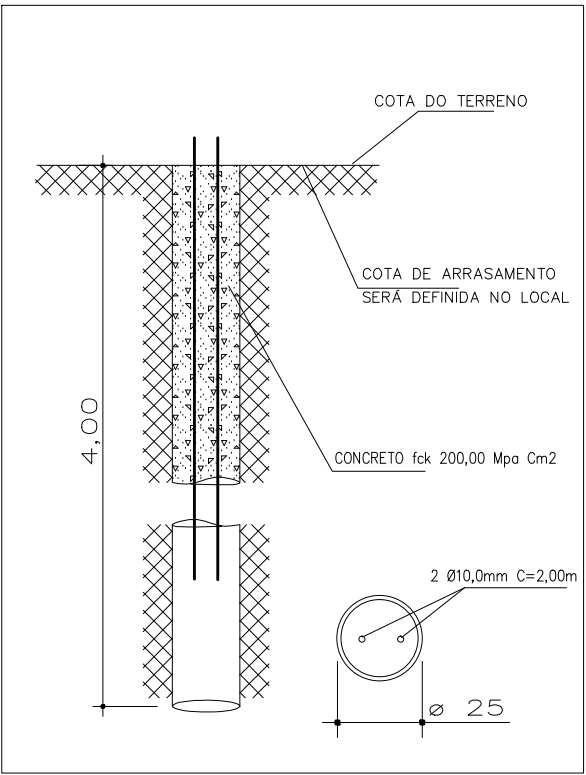
ESTACA Ø 25Cm X 4,00m x 31
