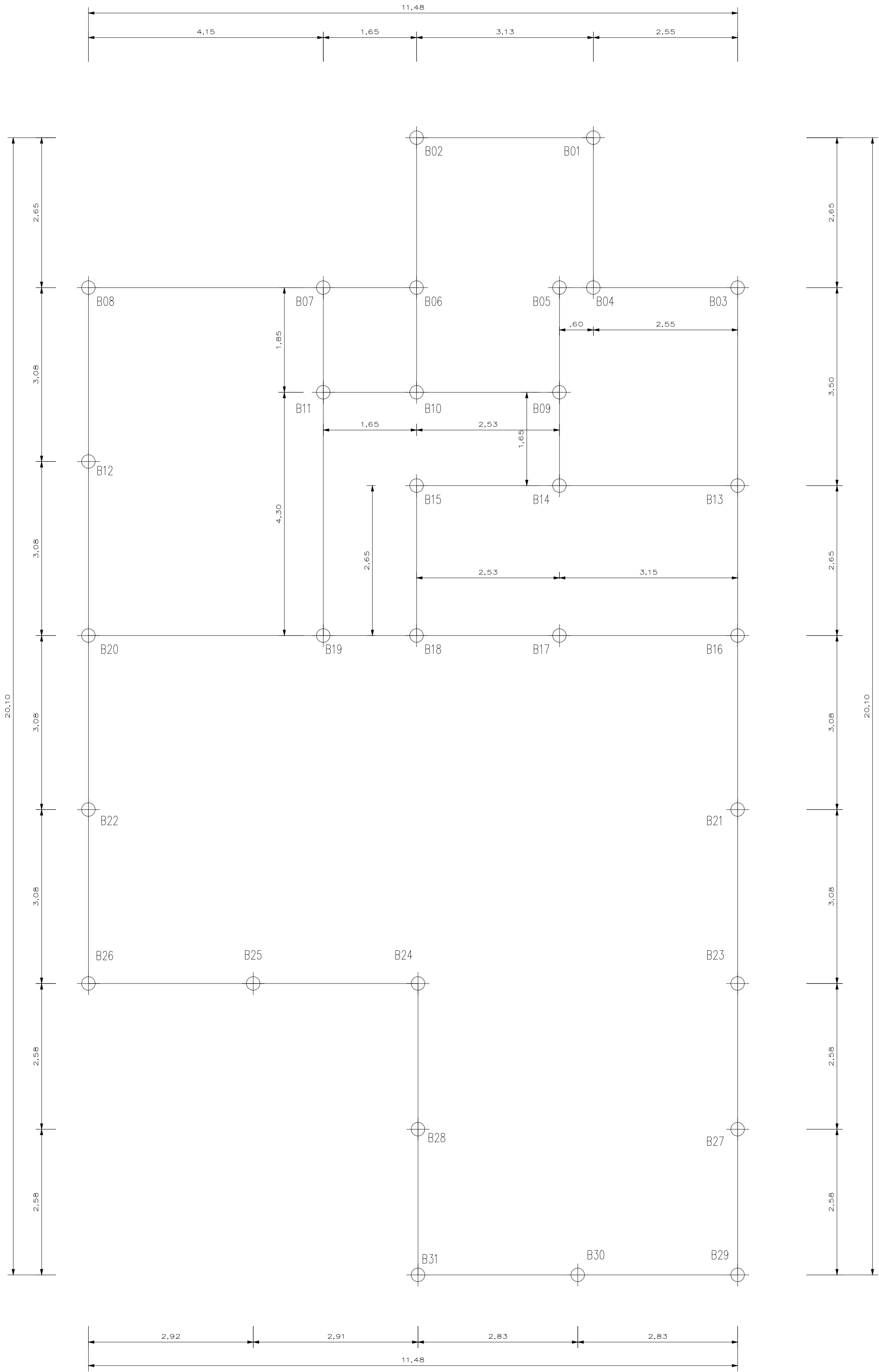
FUNDAÇÃO E LOCAÇÃO DAS ESTACAS – ESC. 1/50
