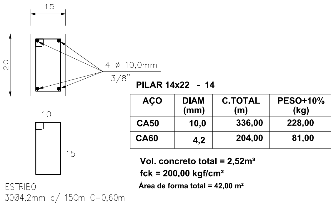
PILAR SECÃO TRANSVERSAL ESCALA 1/10
