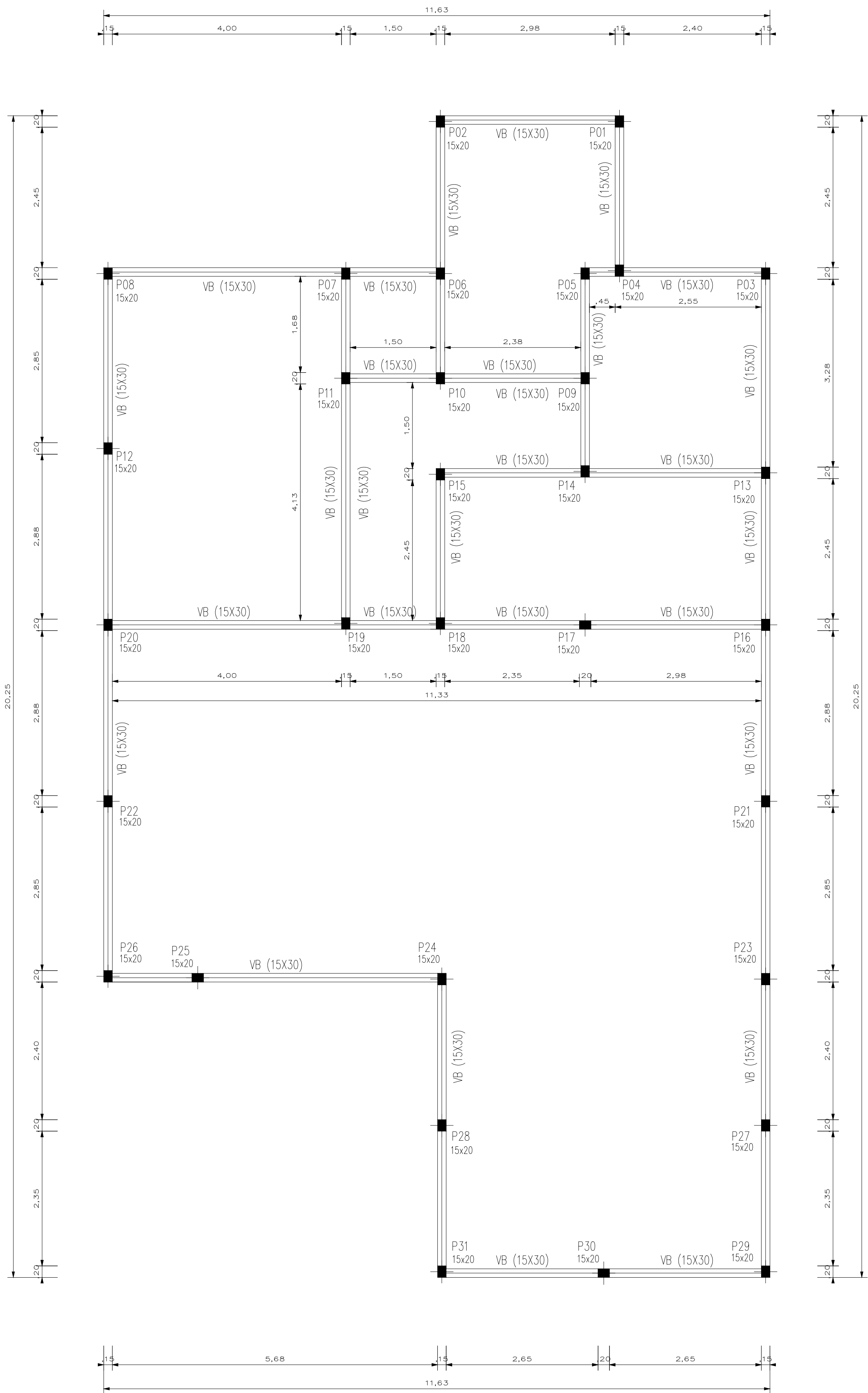
PLANTA DE FORMAS DAS VIGAS –BALDRAMES – PILARES – ESC. 1/50
